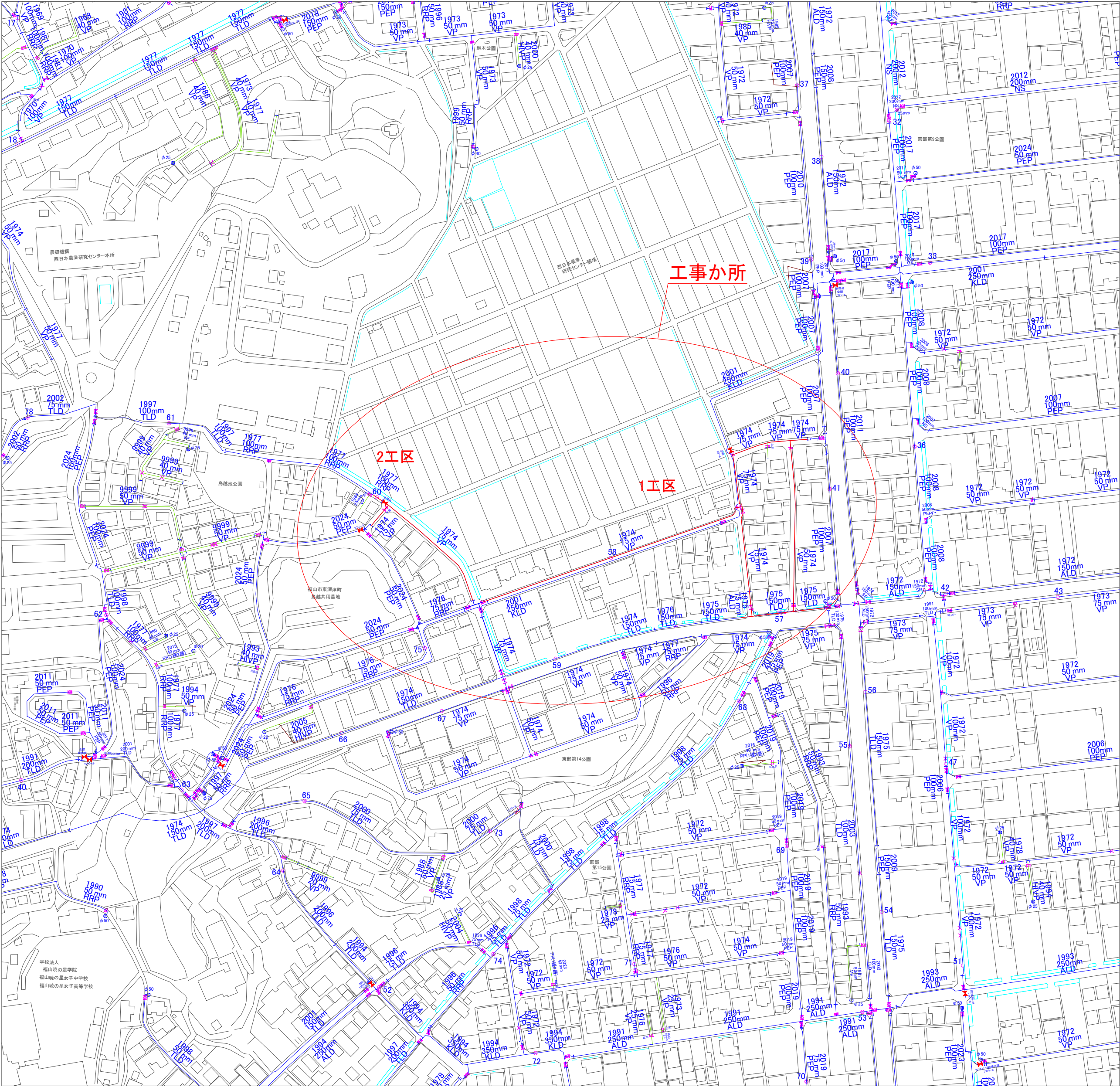
配管図 S=1:2500
