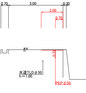
5-5' 断面
