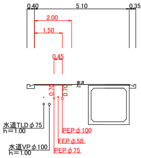
4-4' 断面
