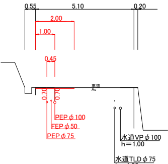
3-3' 断面
