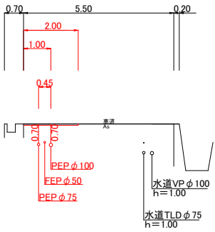
1-1' 断面
