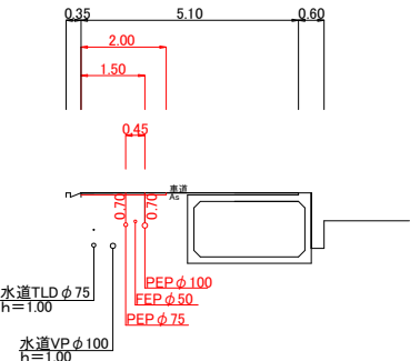
2-2' 断面
