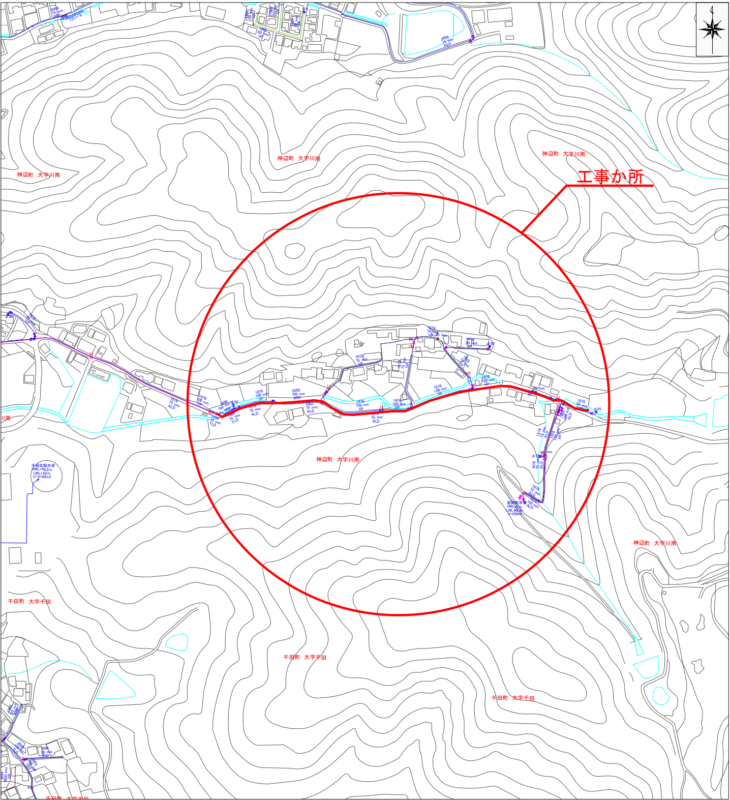
配管図 S=1／2500
