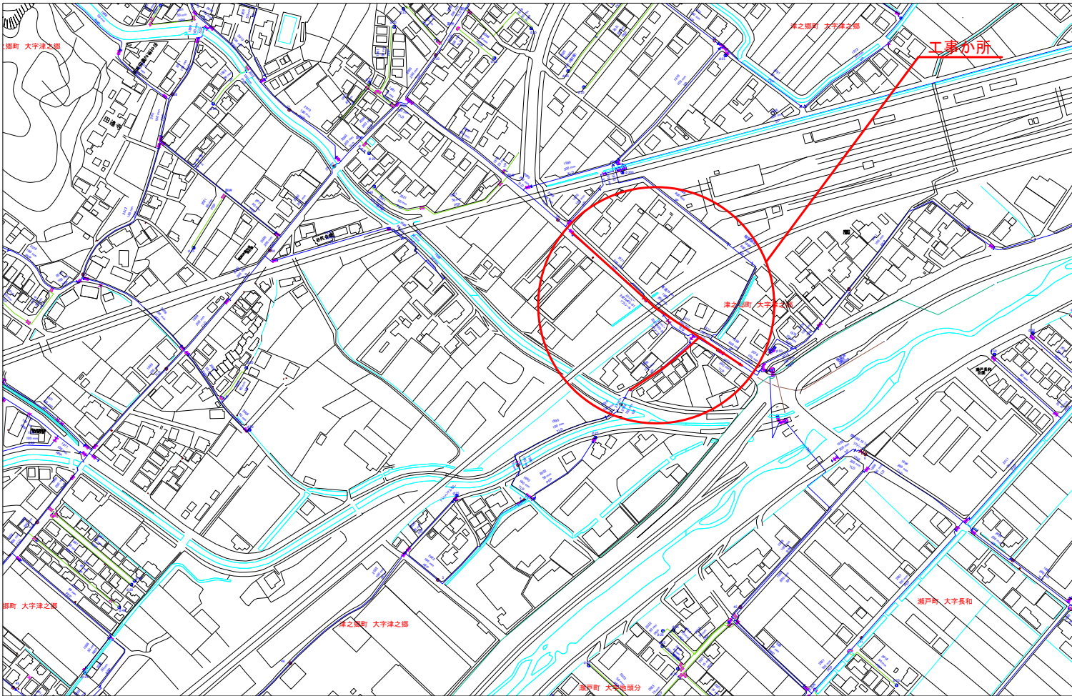
配管図 S=1/2500
