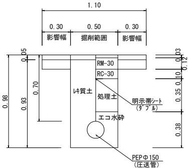
土工断面図 S=1/20
