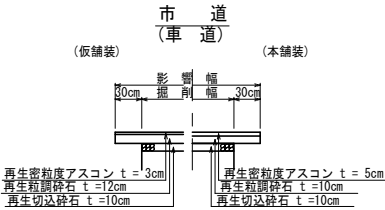
舗装断面図 S=1/50
