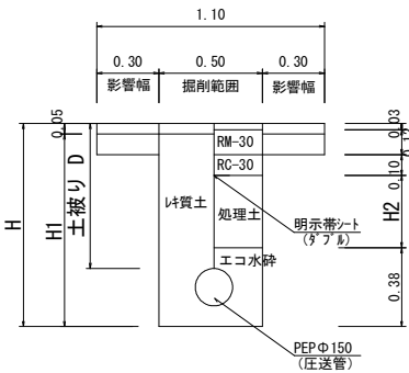
土工断面図 S=1/20
