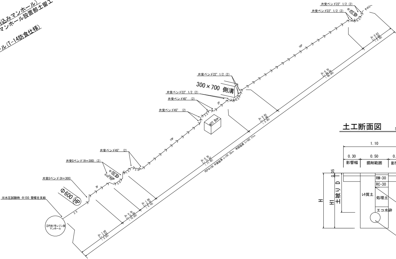
圧送管詳細図 S=Non (その1)
