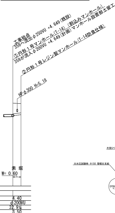
管渠埋設縦断面図 S=縦1/100 横1/500
