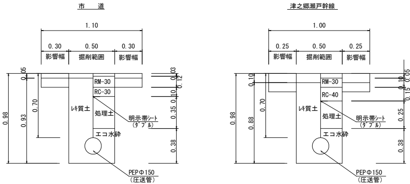
土工断面図 S=1/20
