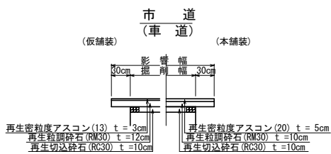
舗装断面図 S=1/50
