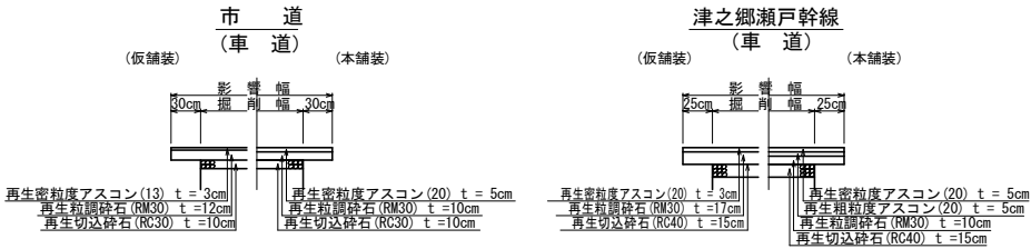
舗装断面図 S=1/50
