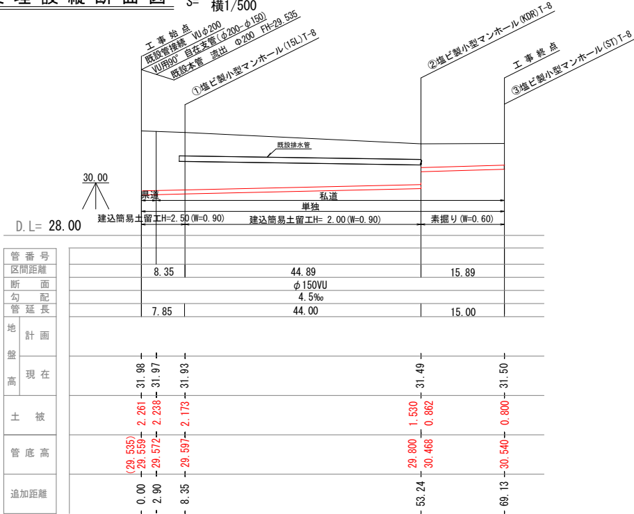
管渠埋設縦断面図 S= 縦1/100 横1/500
