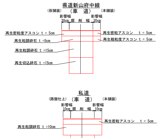
舗装復旧断面 S=1/10
