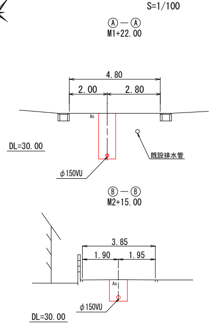
標準断面図 S=1/100
