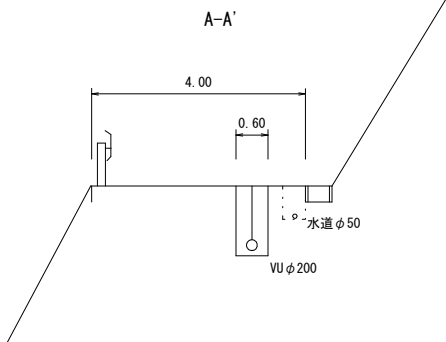
標準横断面図 S=1：100
