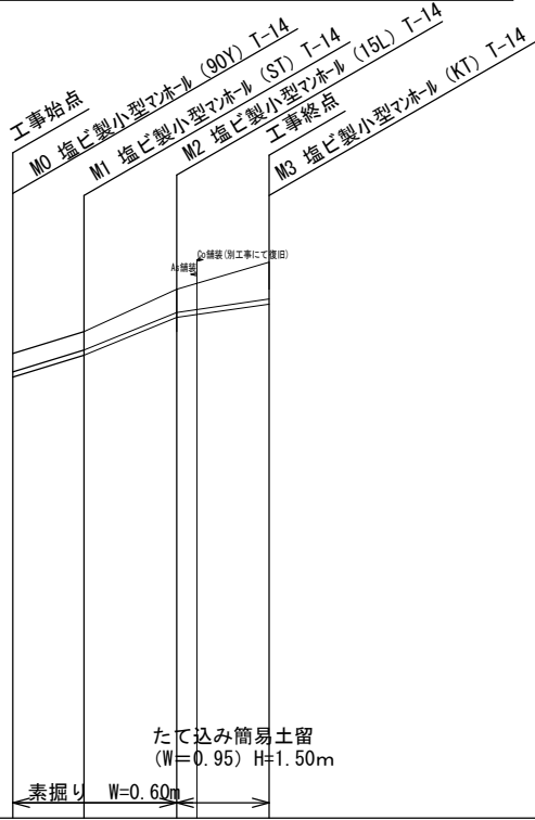
管 渠 埋 設 縦 断 面 図 縦1/250 横1/1000
