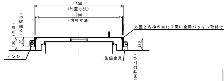
人孔蓋断面図 S=NON
