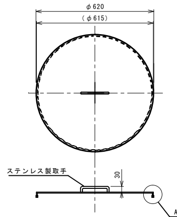
樹脂蓋（塩ビ製）平面図 S=NON
