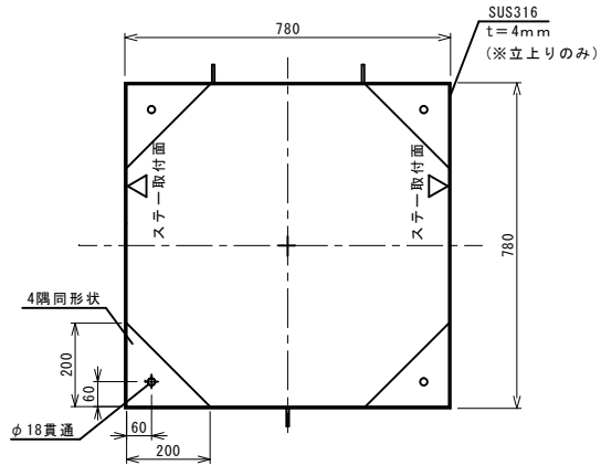
内枠平面図 S=NON
