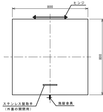
外蓋平面図 S=NON
