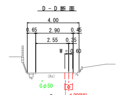
舗装復旧断面図 S=1/10
