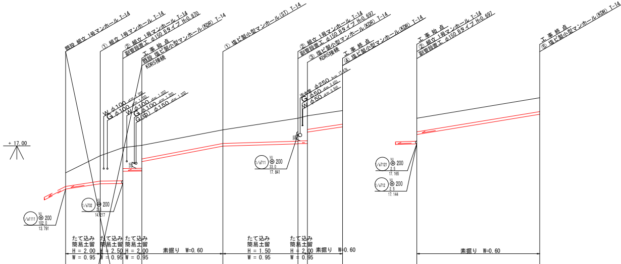
管渠埋設縦断面図 S=縦1:100 横1:500
