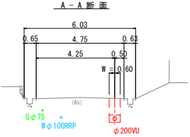
管渠埋設断面図 S=1:100
