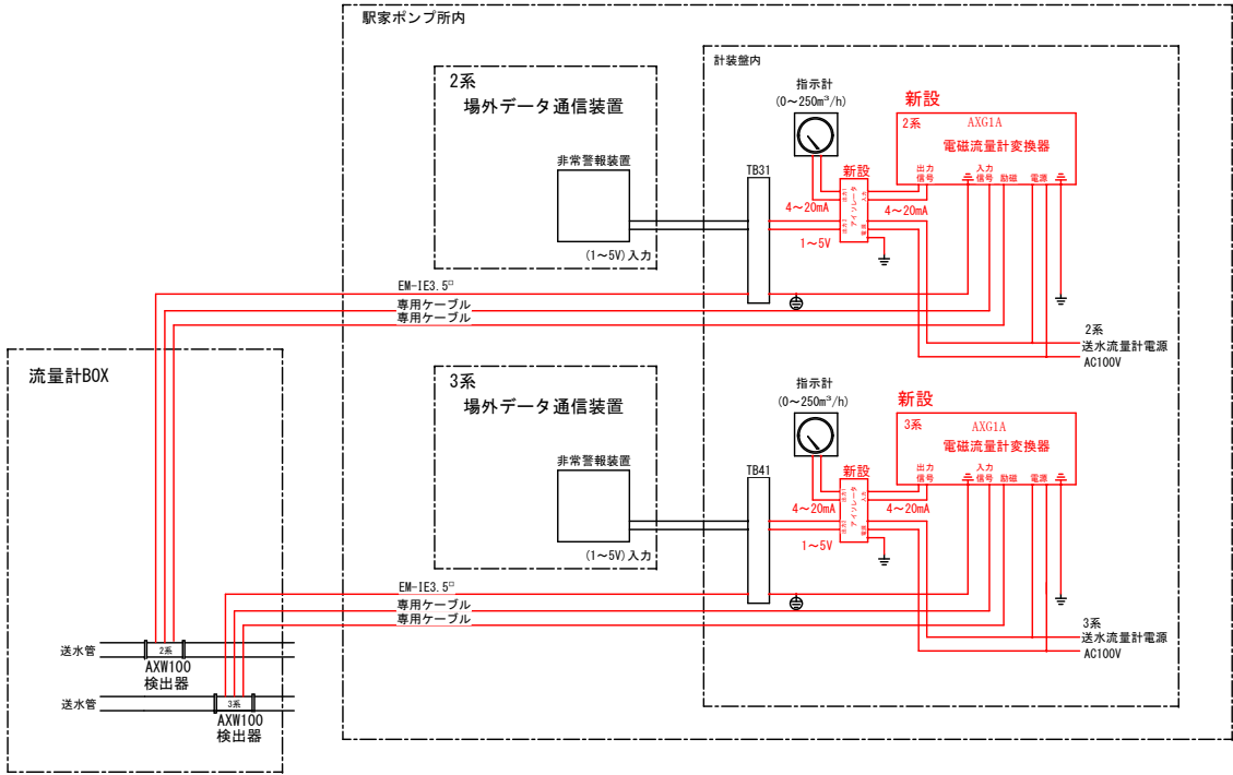
新設図面 赤線部新設
