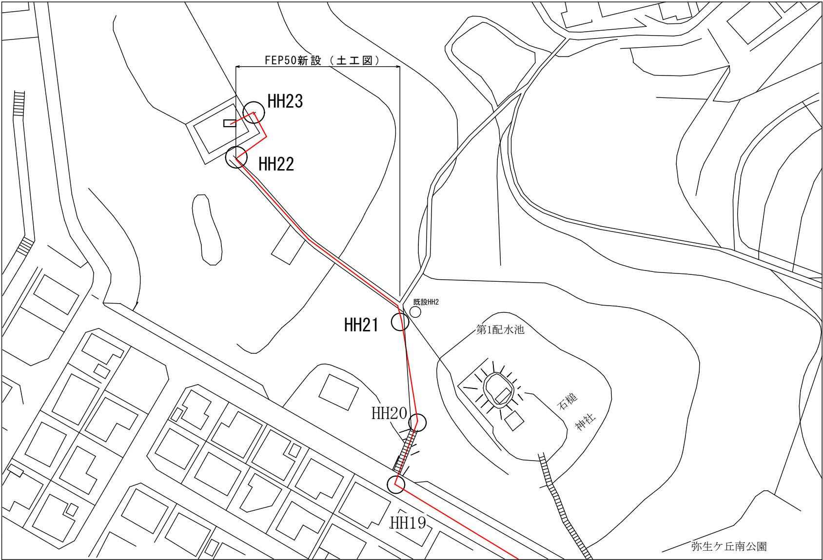
配水池 周辺図
