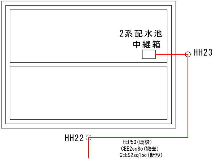
配水池平面図
