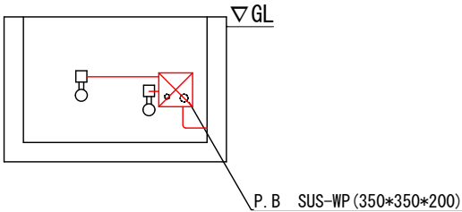
A-A' 断面図
