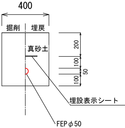
土工図
