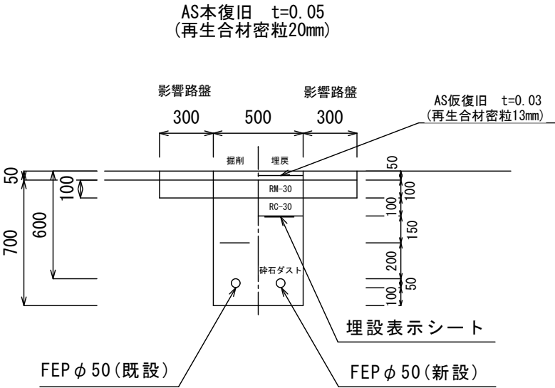
土工図 (S=1/30)
