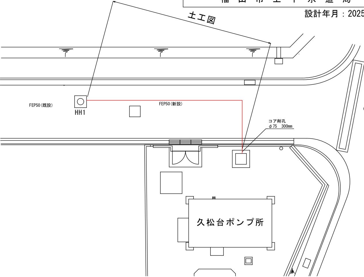
久松台ポンプ所 平面図
