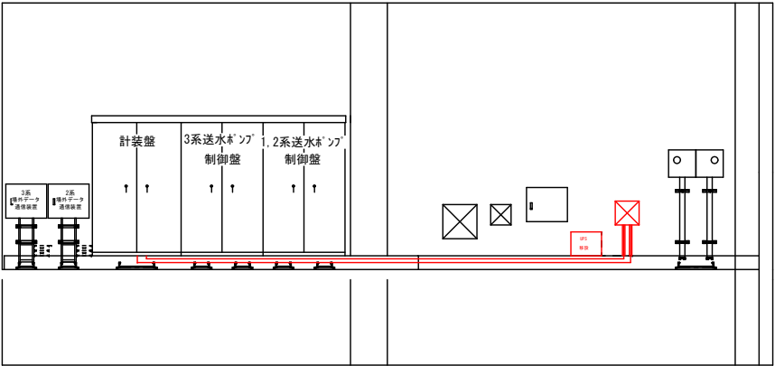
ポンプ室側面図
