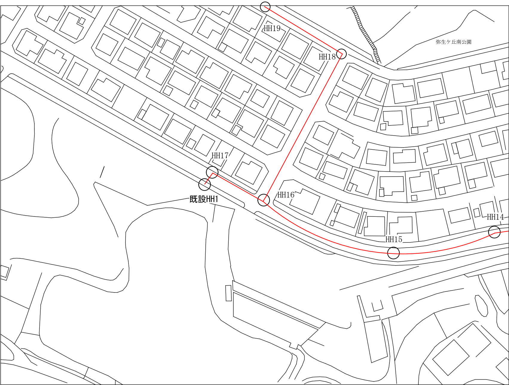
中間地点 平面図
