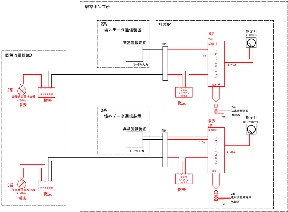
撤去図面 赤線部撤去
