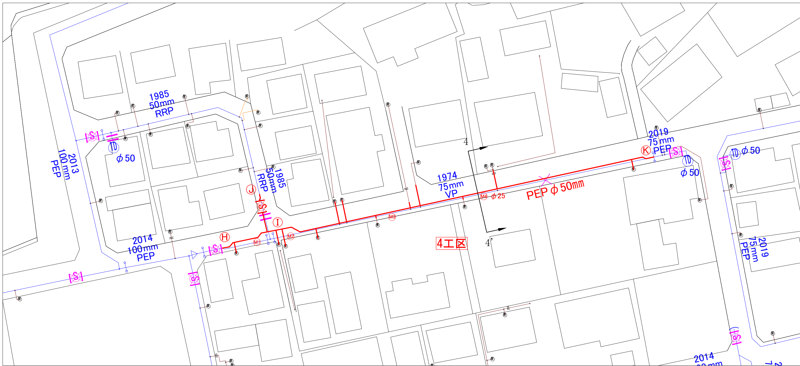
平面図(4工区) S=1/500
