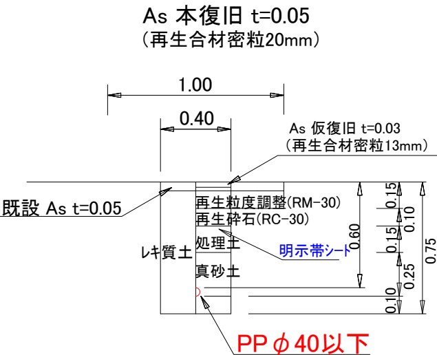
給水管φ40土工図
