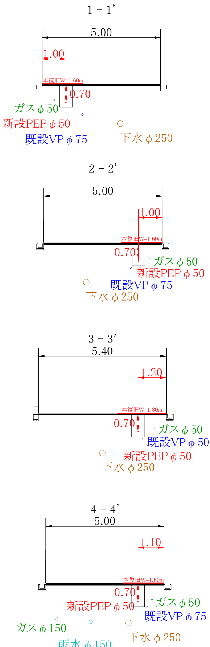
横断面図(1~4工区) S=1/100
