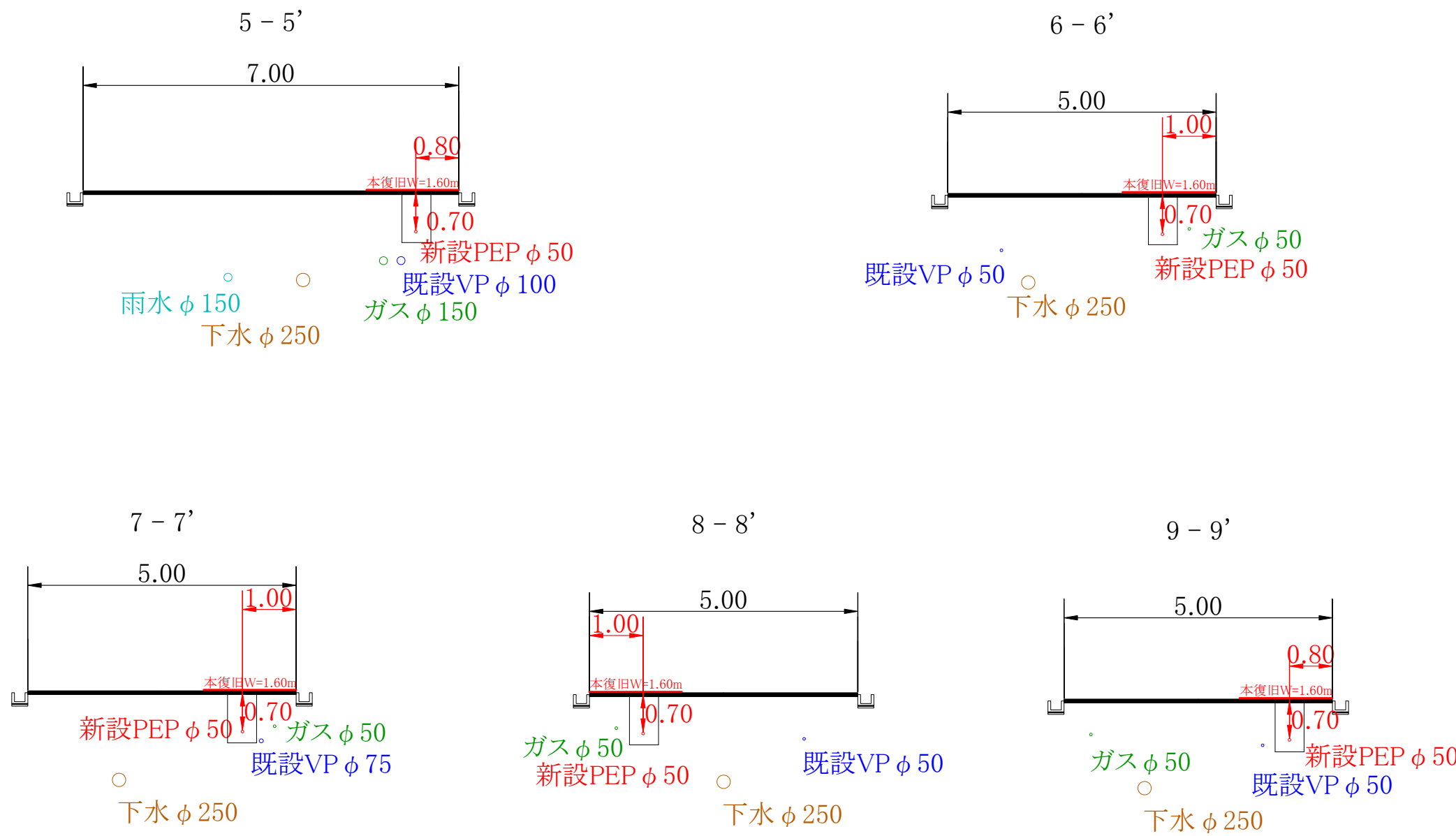
横断面図(5～7工区)
