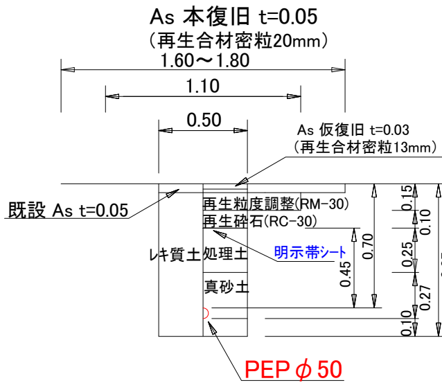
PEP・ドレンφ50土工図
