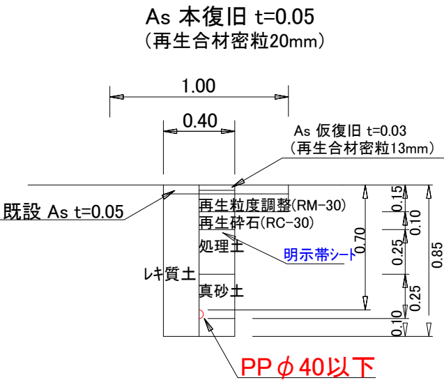
給水管φ40土工図
