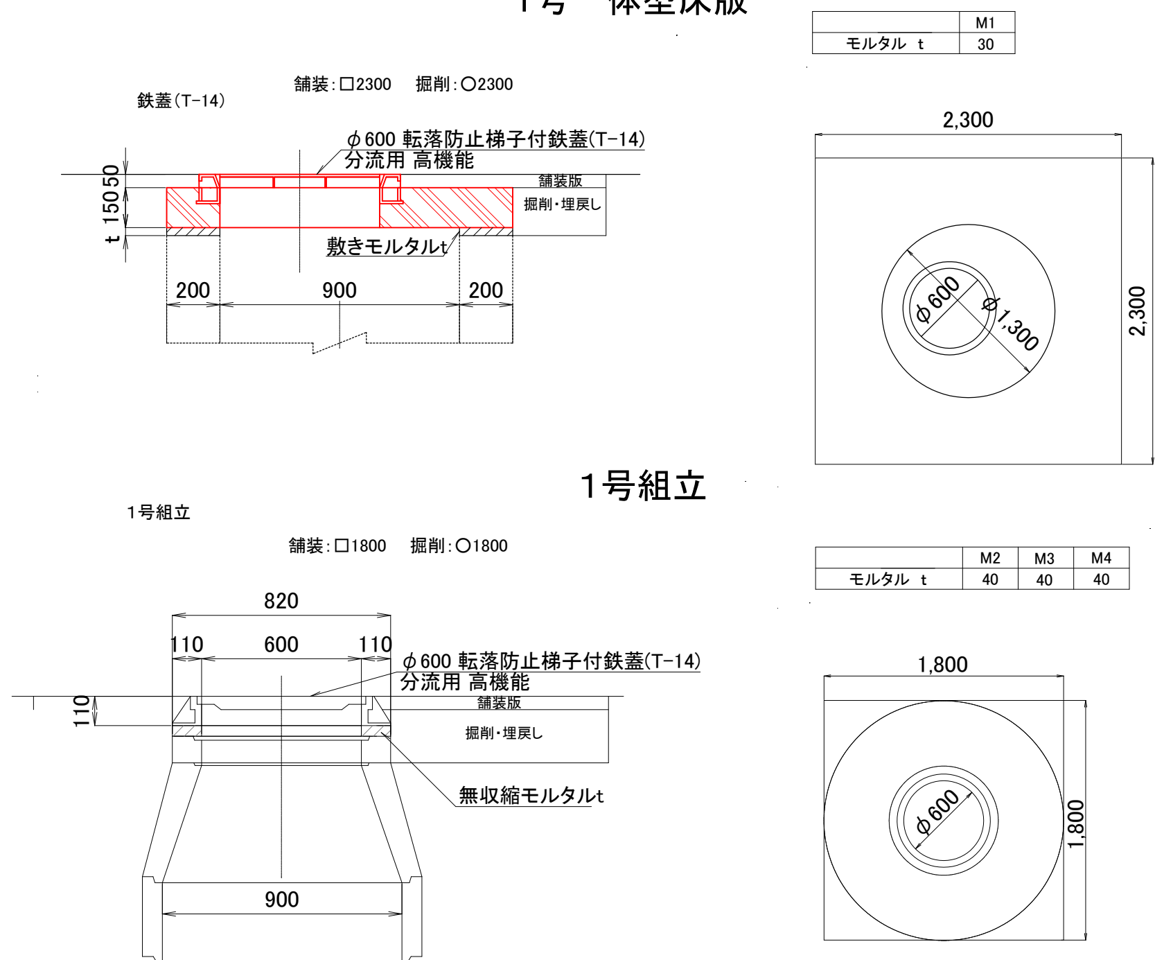
マンホール蓋取替標準図 S=NON
