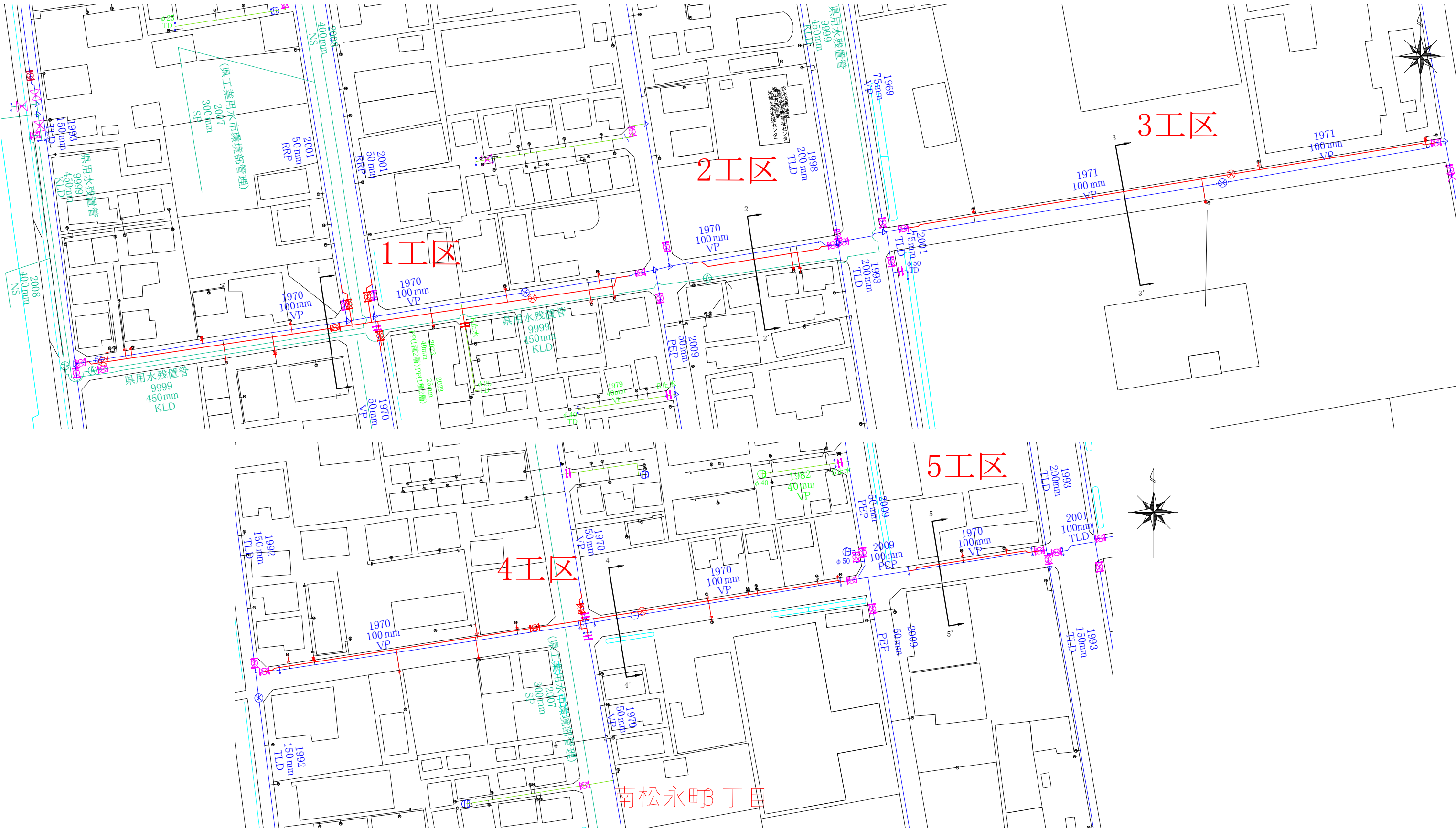
平面図 S=1/600
