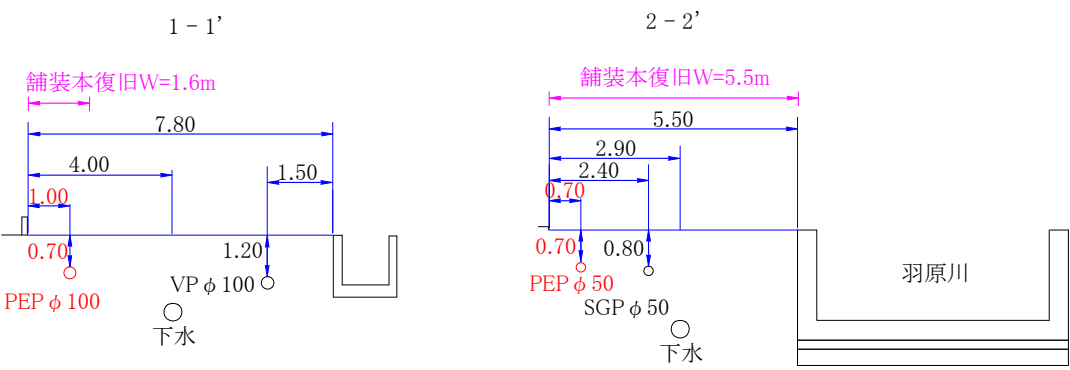
横断面図 S=1/100
