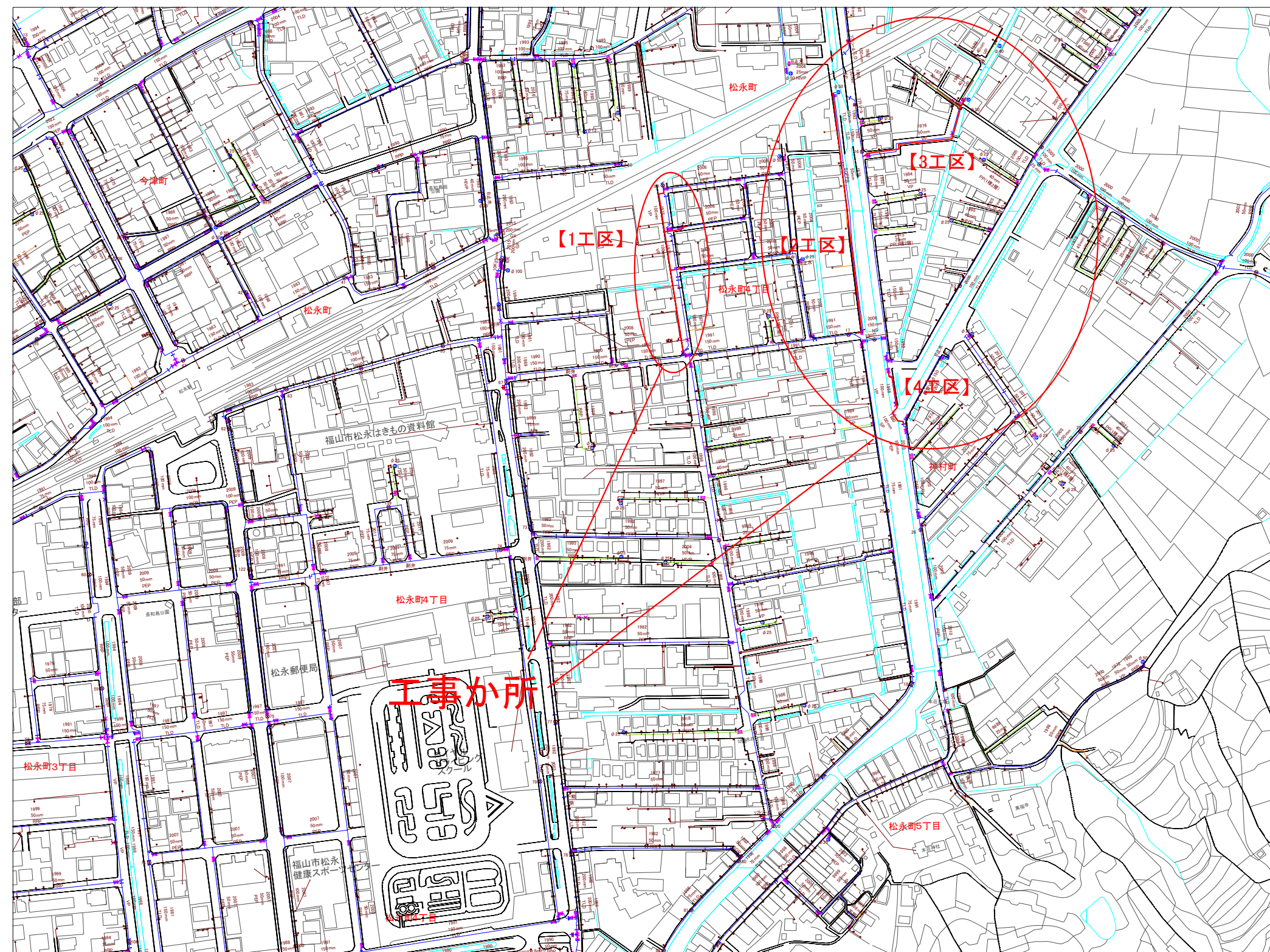
配管図 S=1/2500
