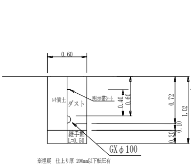
(農道路肩部) 給水管GXφ100土工図⑦
