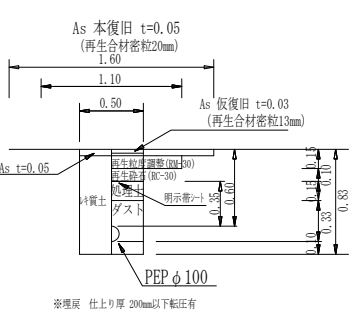
(農道車道部) 給水管PEPφ100土工図⑧
