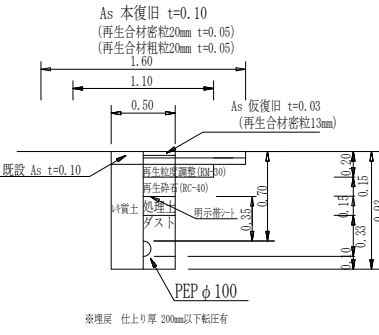
(市道車道部) PEPφ100土工図③ 給水管PEPφ100土工図⑤
