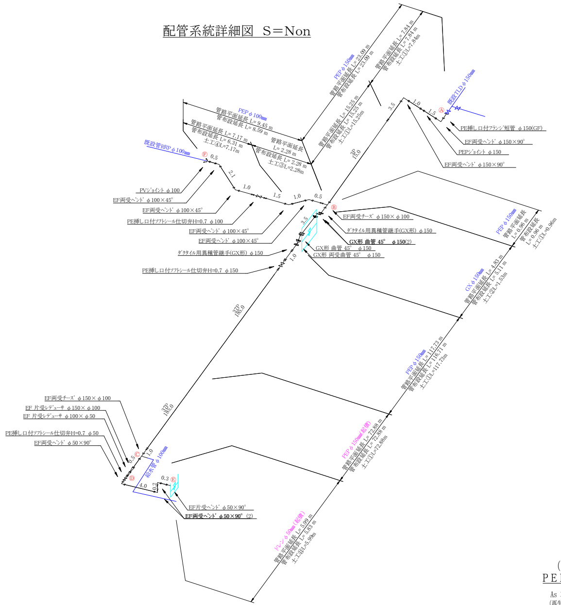
【給水管φ100mm】配管系統詳細図 S=Non
