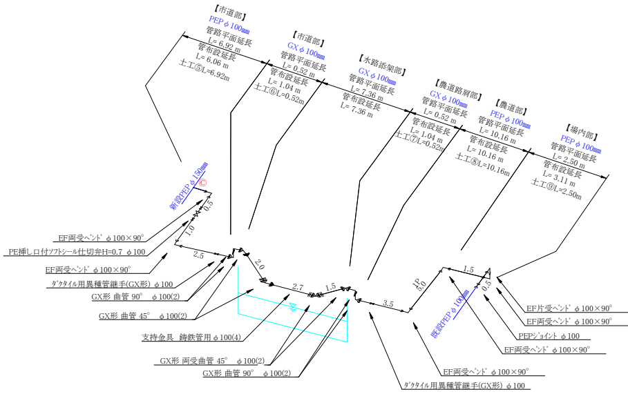
【給水管φ100mm】配管系統詳細図 S=Non
