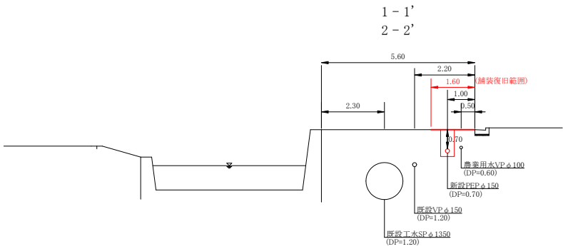
横断面図 S=1/100
