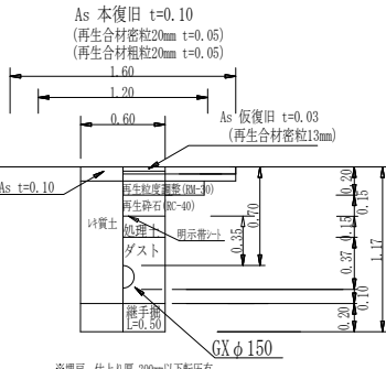
(市道車道部) GXφ150土工図②
