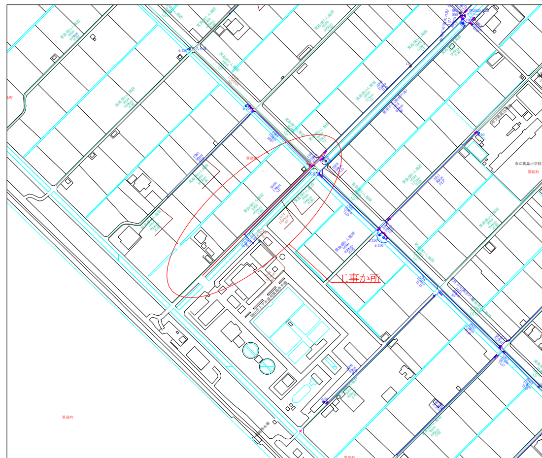
配管図 S=1/2,500
