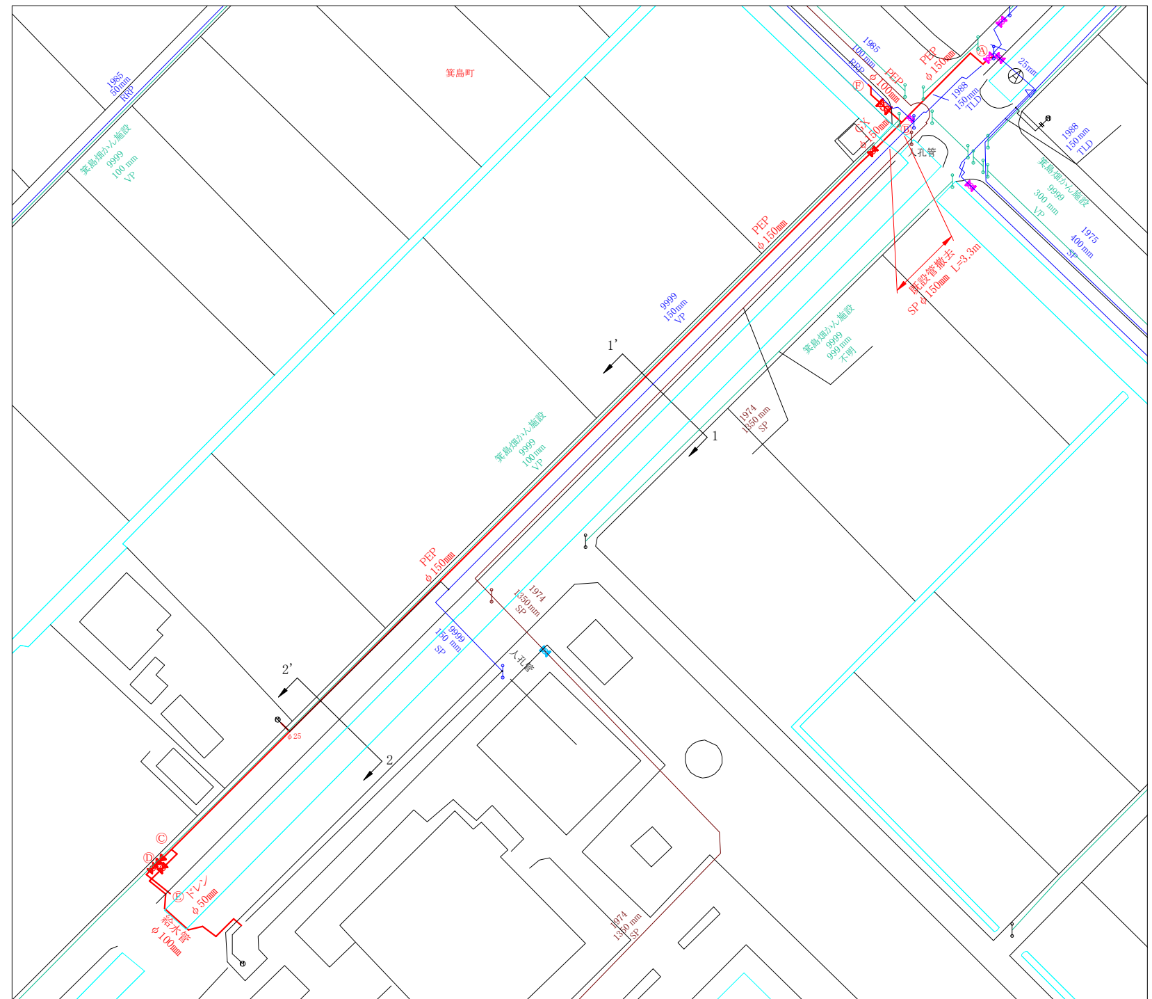
平面图 S=1/500
