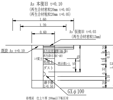
(市道車道部) 給水管GXφ100土工図⑥
