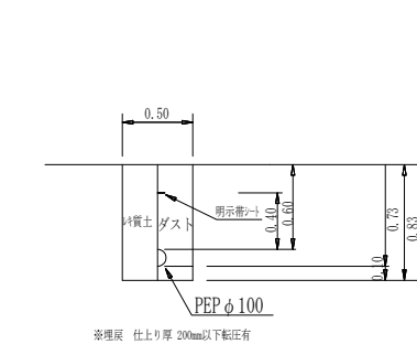
(浄水場場内) 給水管PEPφ100土工図⑨
