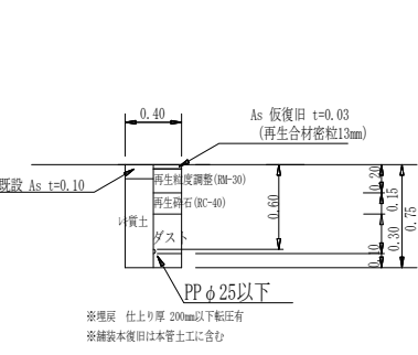
給水管φ25以下土工図⑩
