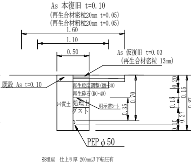
ドレンφ50土工図⑪
