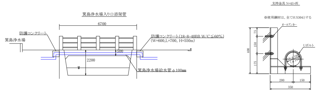
水路断面図 S=1/100
