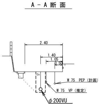
横断面図 S = 1:100
