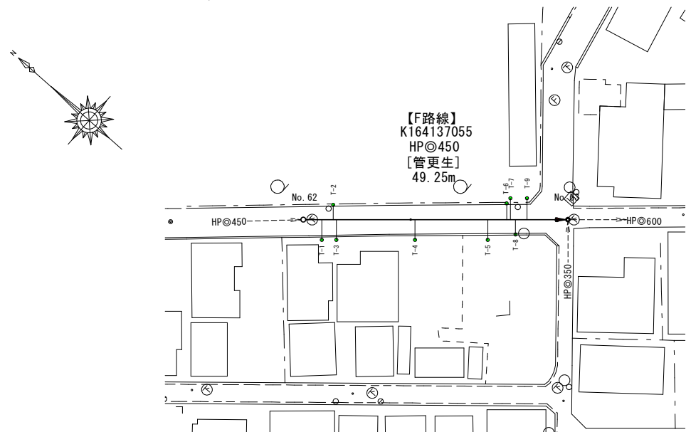
平面図 S=1/500
