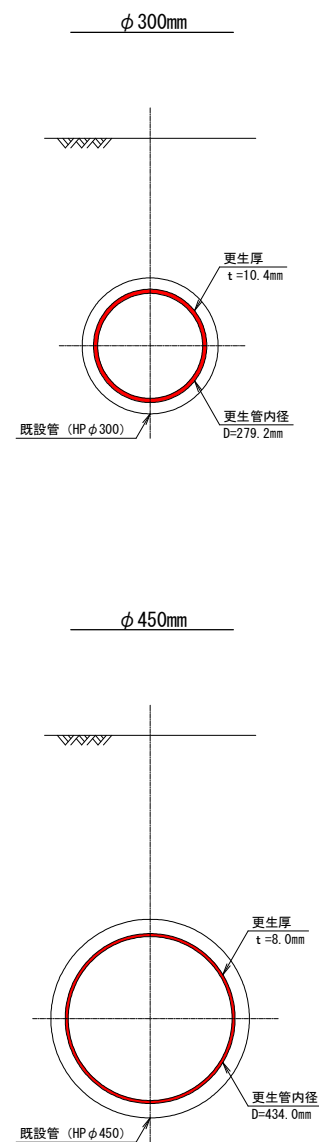
更生断面図（参考） S=Free
