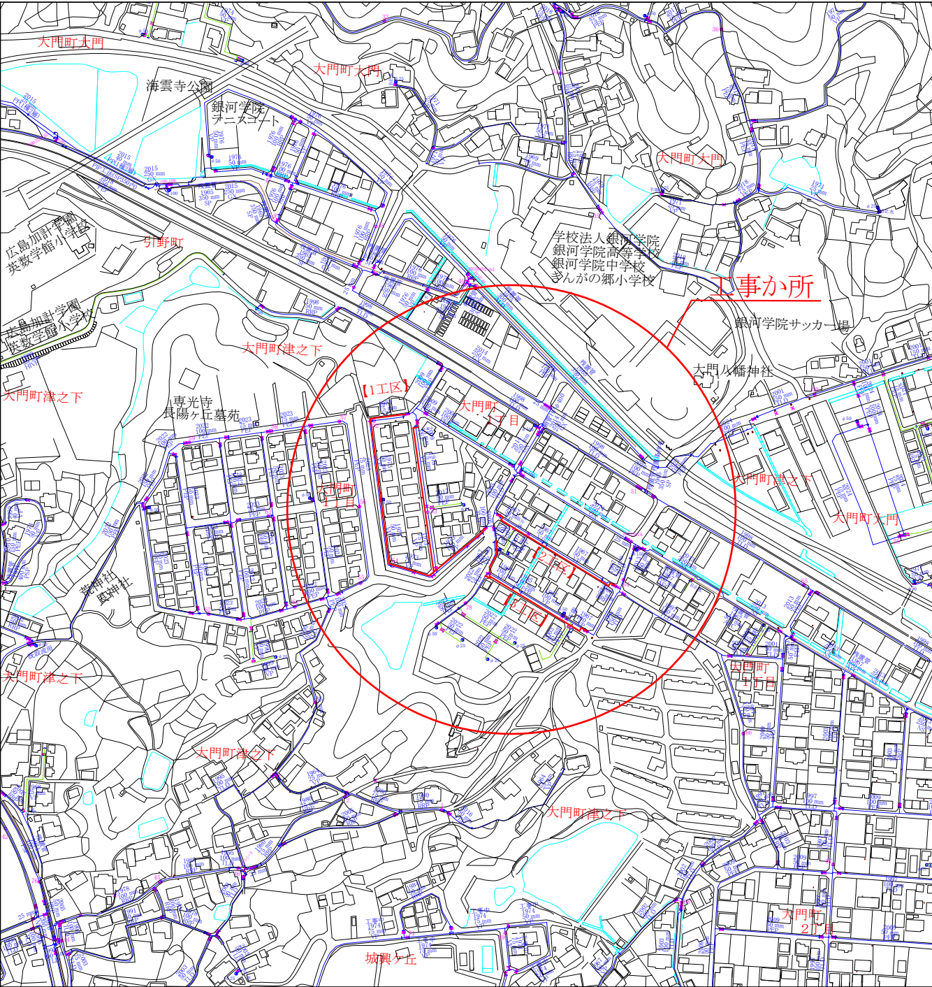
配管図
