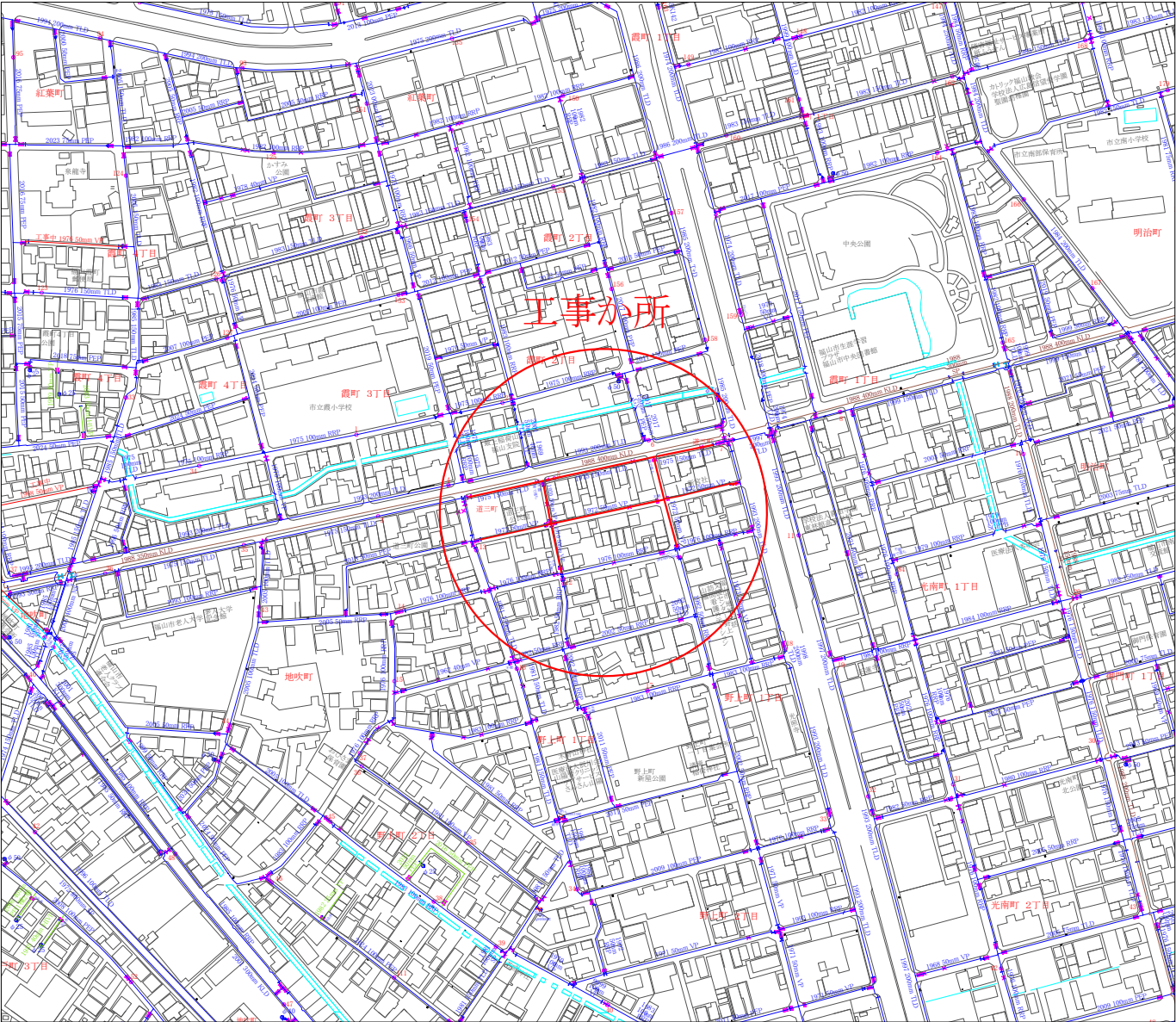
配管図 S=1/2,500
