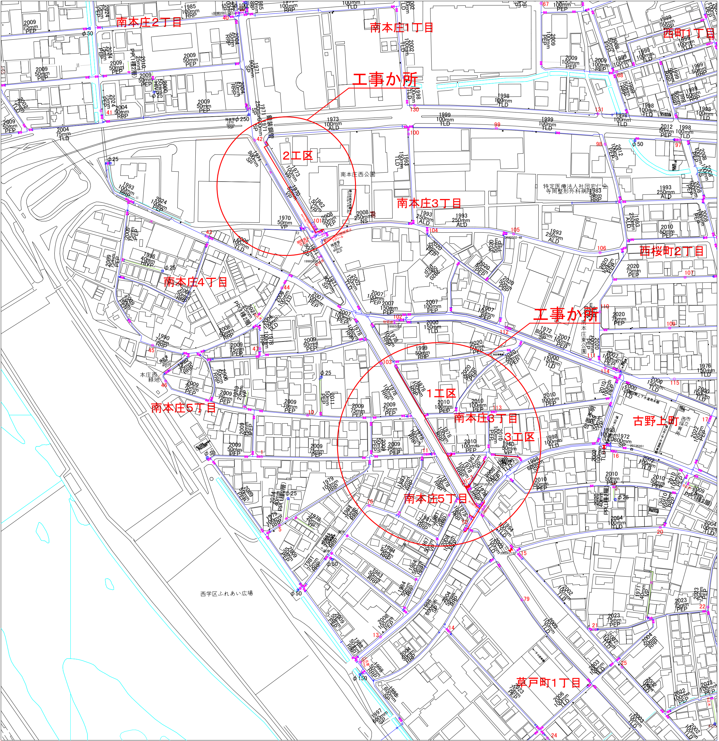
配管図 S=1:2500
