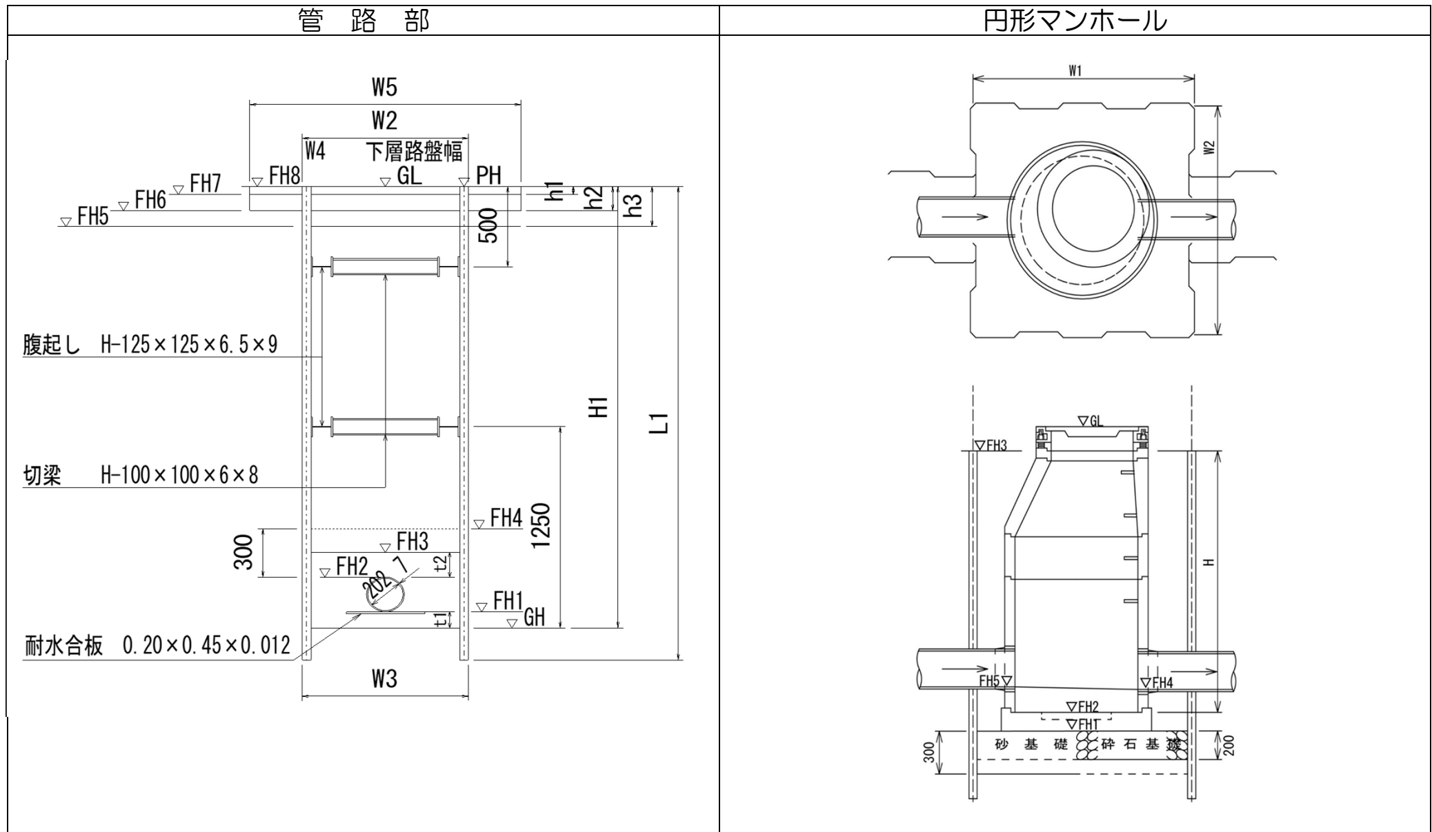
標準図 (1)
