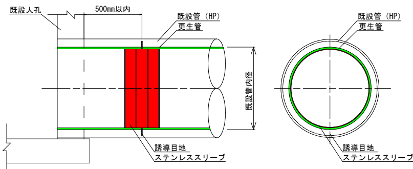
側面図
