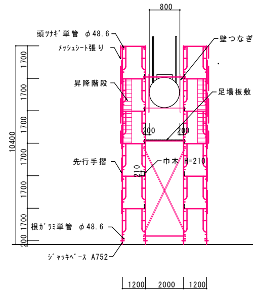
横断面図 1/100
