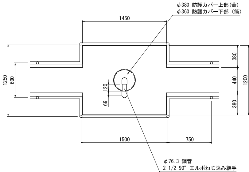
矢視C-C
