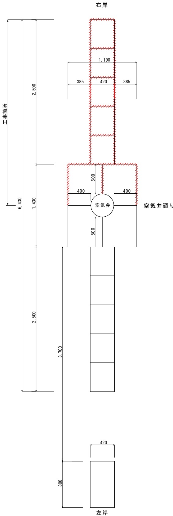
平面図 S=1/200
