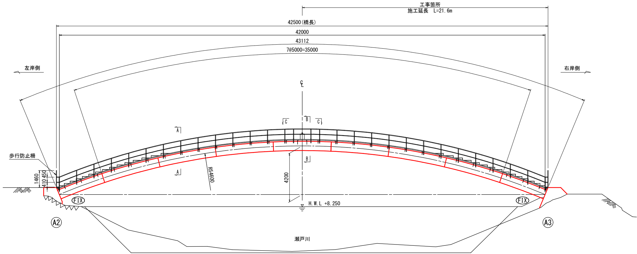
側面図 S=1:100
