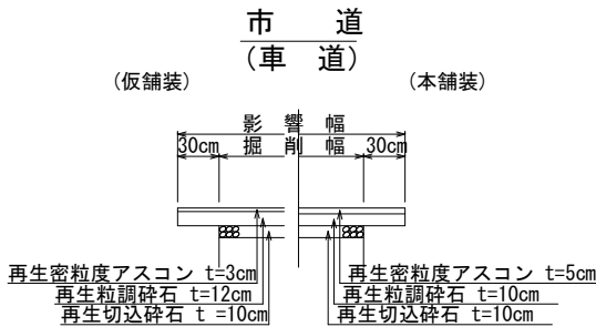
舗装断面図
