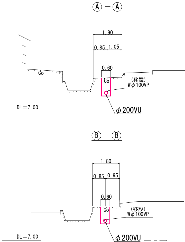
標準横断面図
