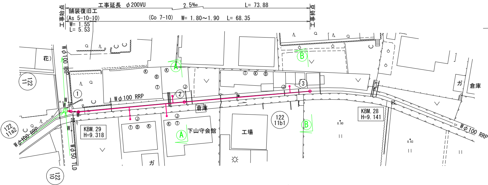
管渠埋設縦断面図
