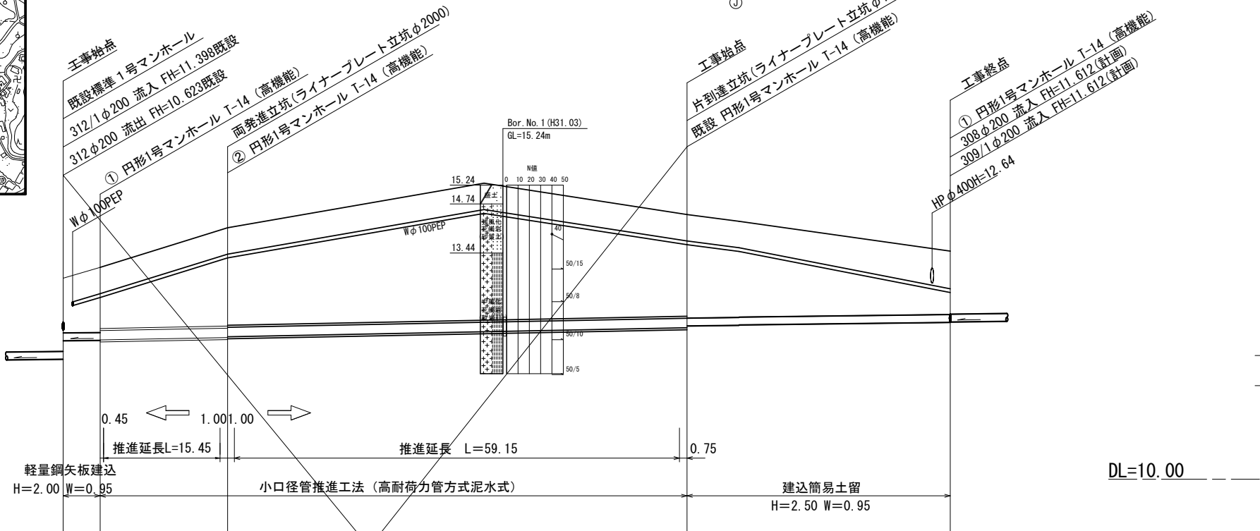
管渠埋設縦断面図 V=1/100 H=1/500
