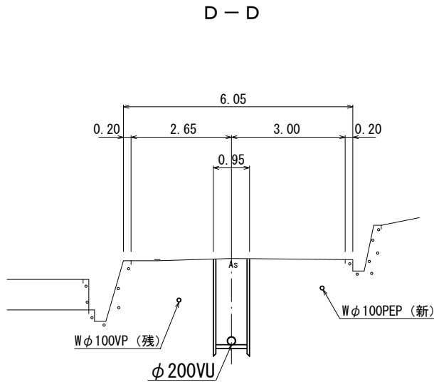
横断面図 S=1/100
