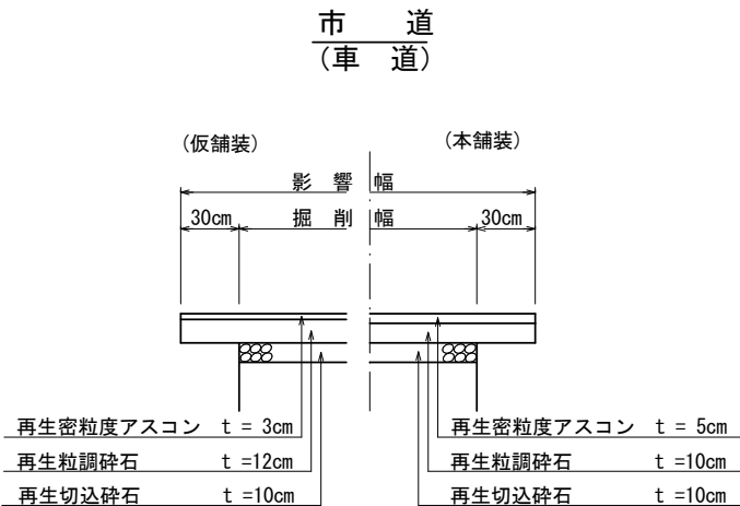
舗装断面図 S=1/30
