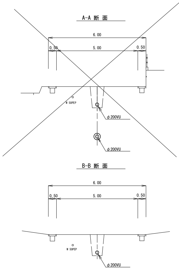
管渠埋設断面図
