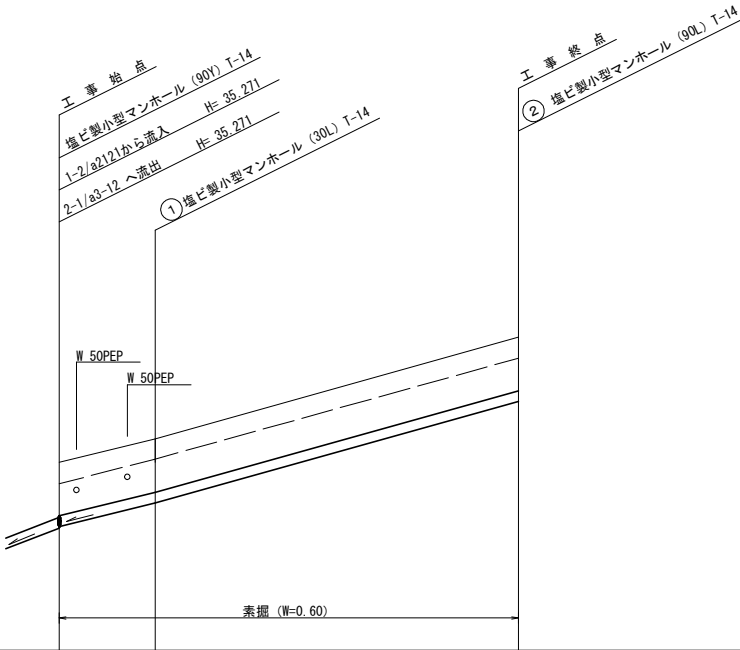
管渠埋設縦断面図
