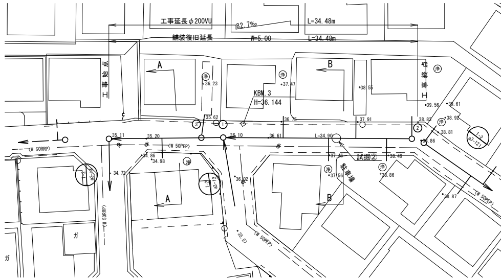
管渠埋設平面図
