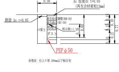
消火栓土工図
