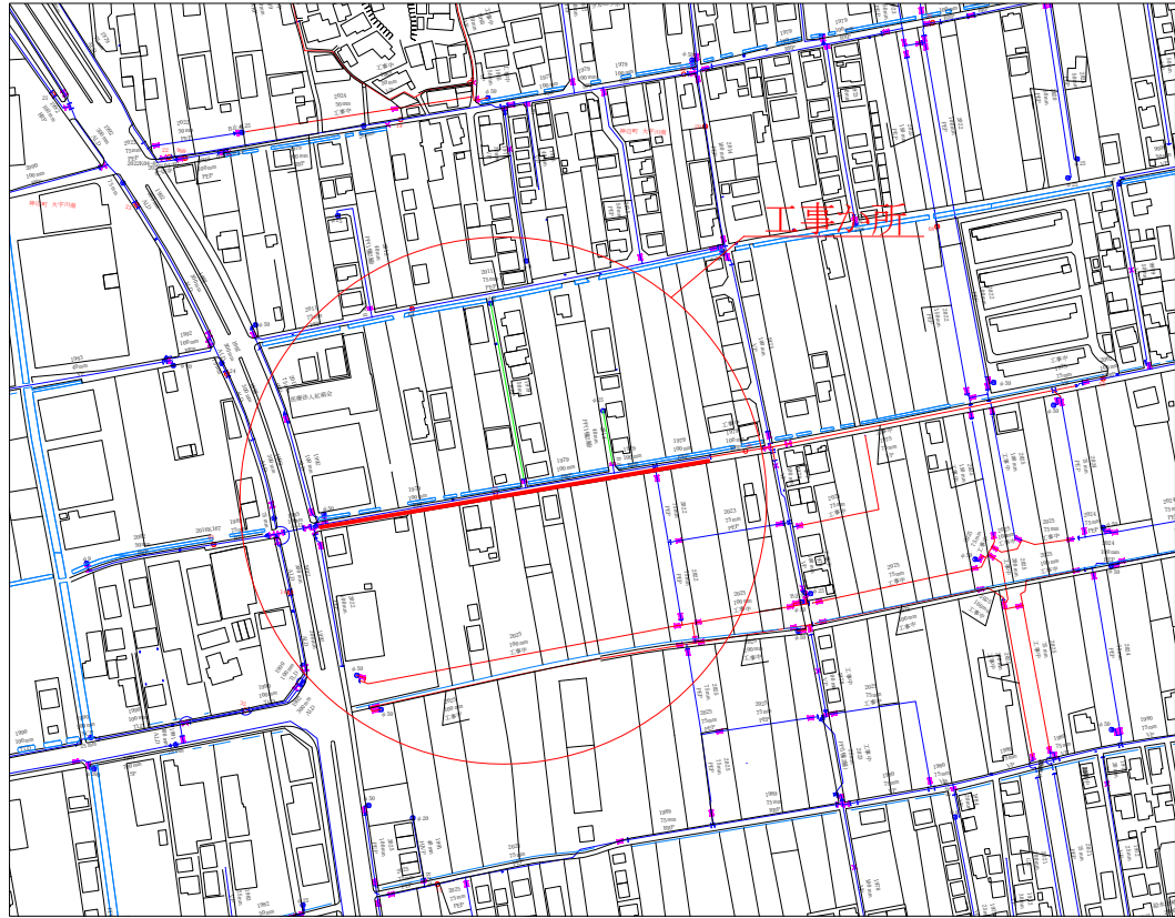
配管図 S=1/2500
