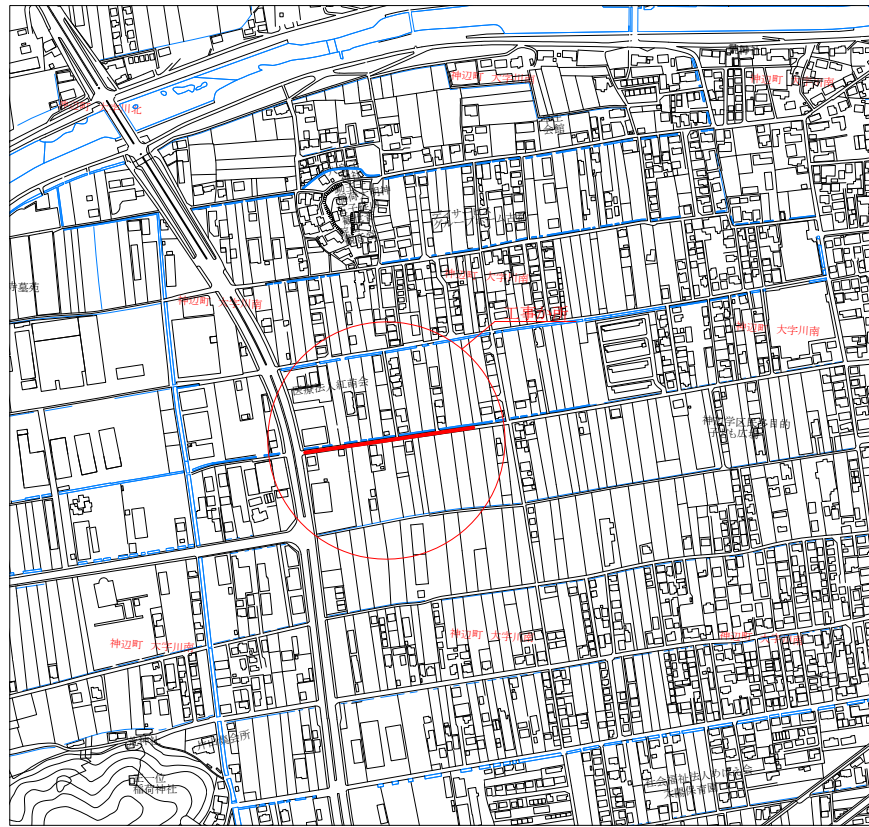
位置図 S=1/5000
