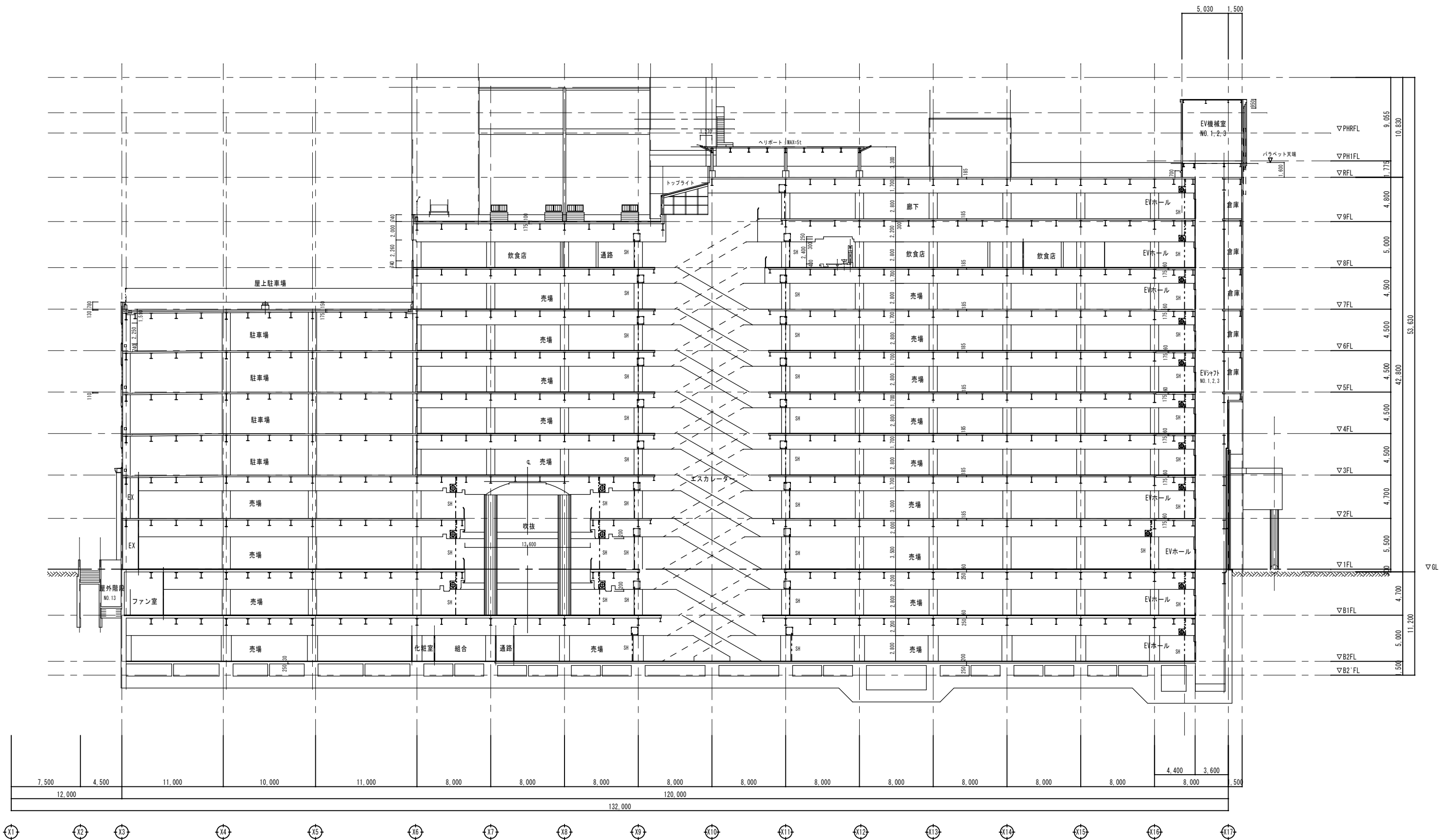
断面図 S=1:200
