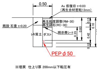
給水管φ50土工図
