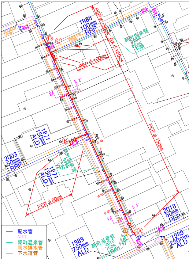
平面図 S=1/500
