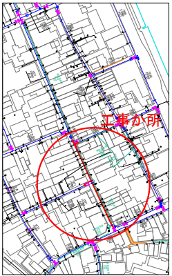
配管図 S=1/2500
