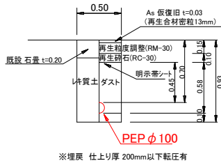
PEPφ100土工図
