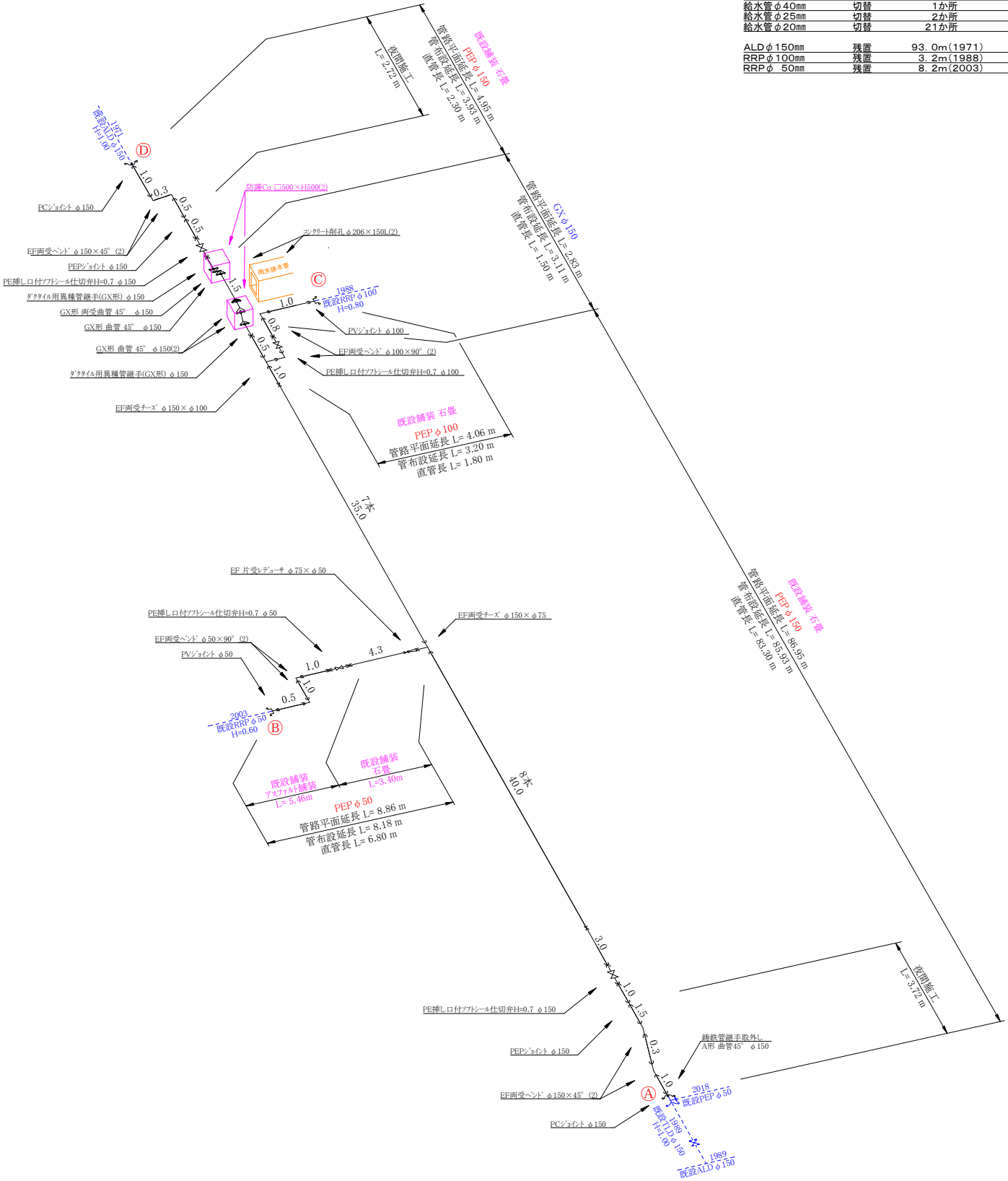
配管系統詳細図 S=non
