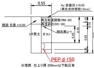
PEPφ150土工図
