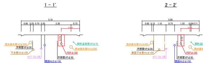
横断面図 S=1/100
