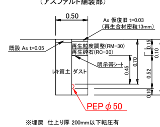
PEPφ50土工図
