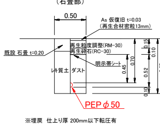
PEPφ50土工図
