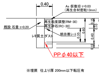
給水管φ40以下土工図
