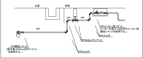
給水管切替標準図 S=non
