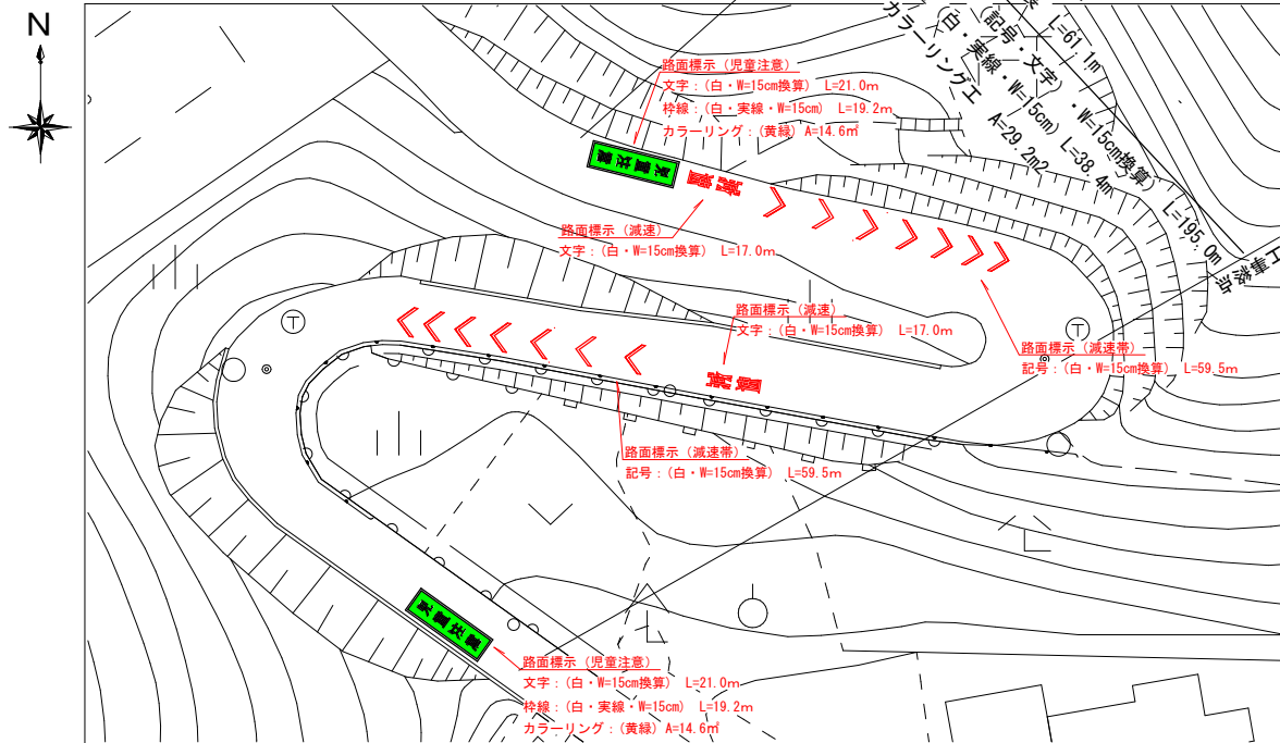
路面標示詳細図
