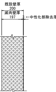
B-B断面図
