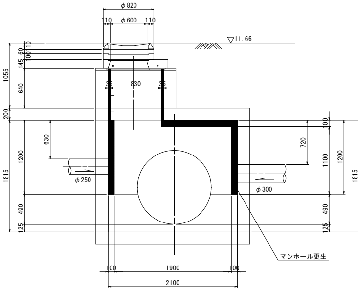
B-B断面図
