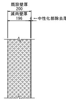
躯体頂版
