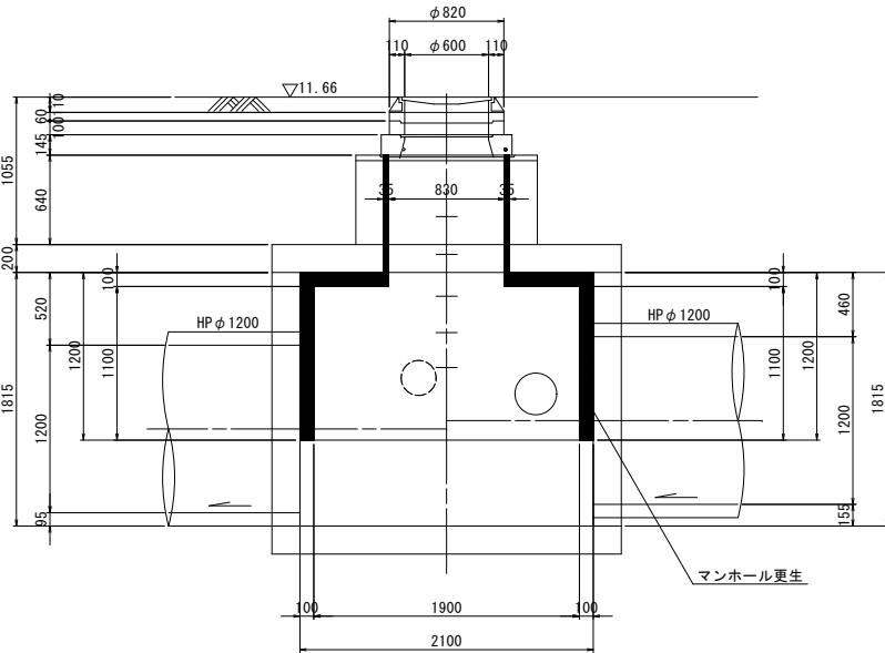
A-A断面図
