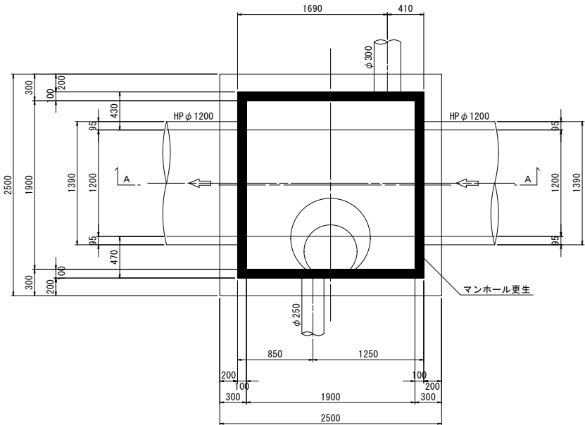
躯体平面図
