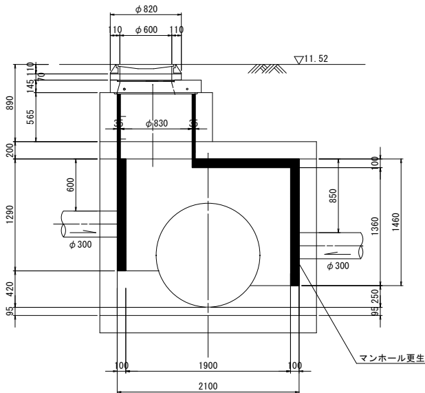
B-B断面図
