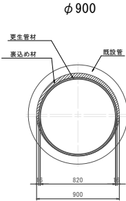
更生管断面図 (参考図面)
