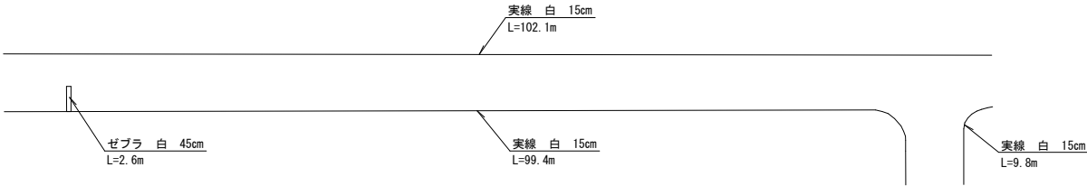
区画線工数量表
