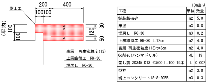
嵩上工 S=1/20
