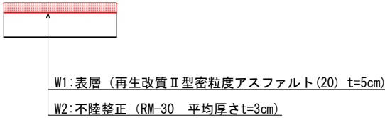
舗装構成 S=1/20
