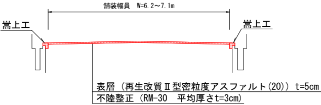
標準横断面図 S=1/100
