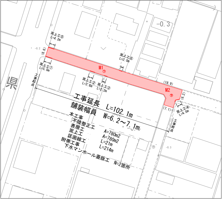
平面図 S=1/1000
