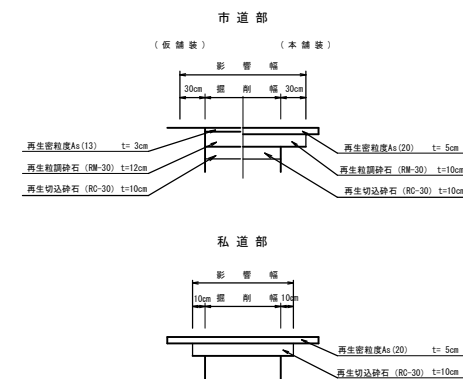
鋪裝復旧断面図 S=1:30
