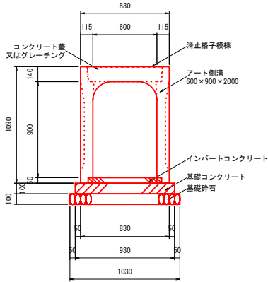
構造図
