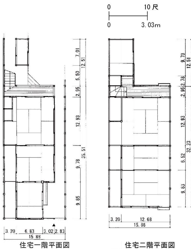
図 1-19 二間半住宅の例
