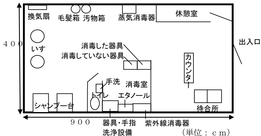
【平面図例】
