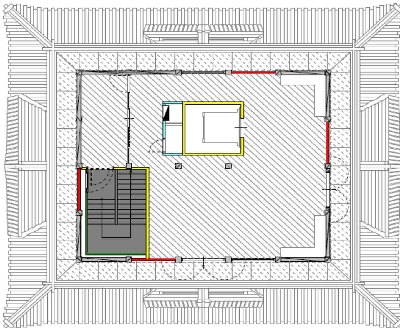
平面図面 福山城天守最上階「天空の間」
