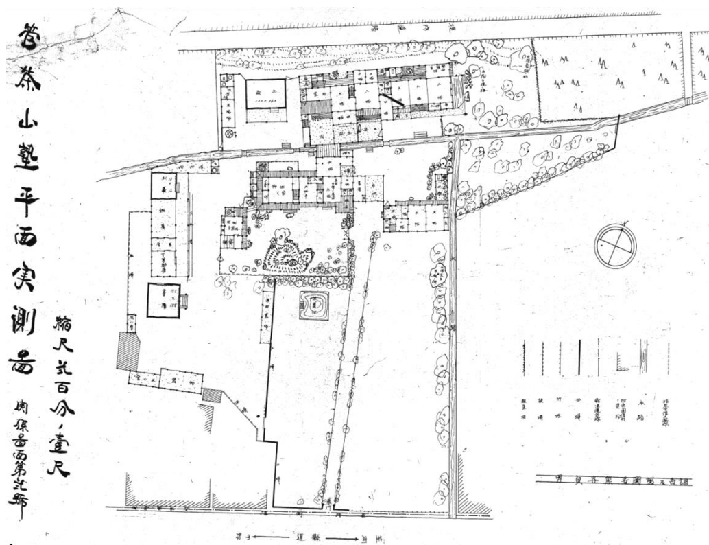
図 3-17 菅茶山塾平面実測図 (1953(昭和 28)年)
