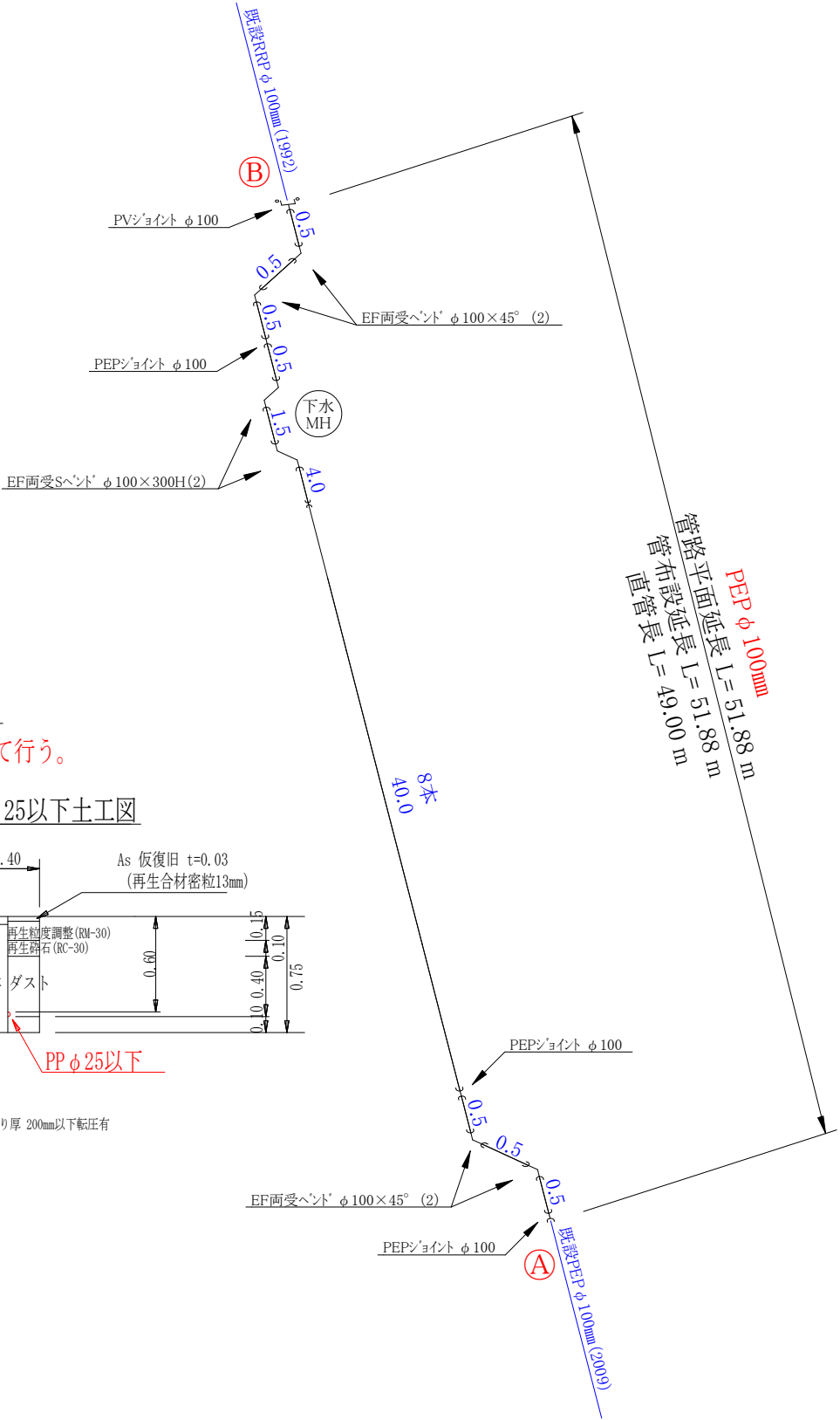
配管系統詳細図 S=NON
