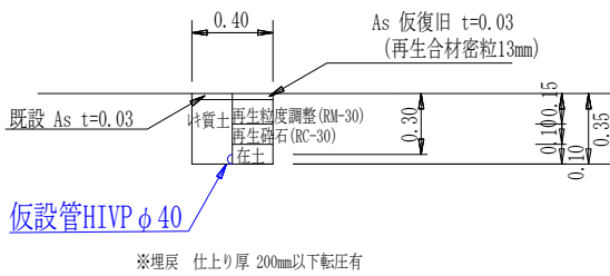
仮設管φ40撤去土工図
