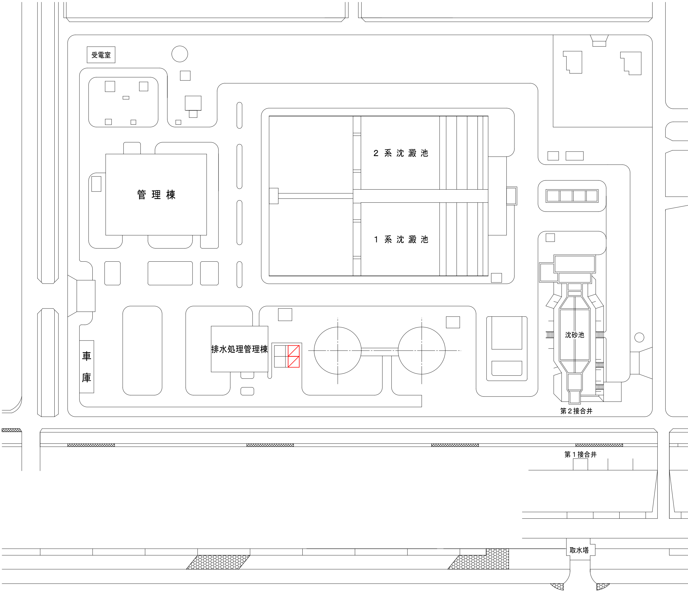
箕島浄水場 配置図 A1:S=1/ 500 A3:S=1/1,000
