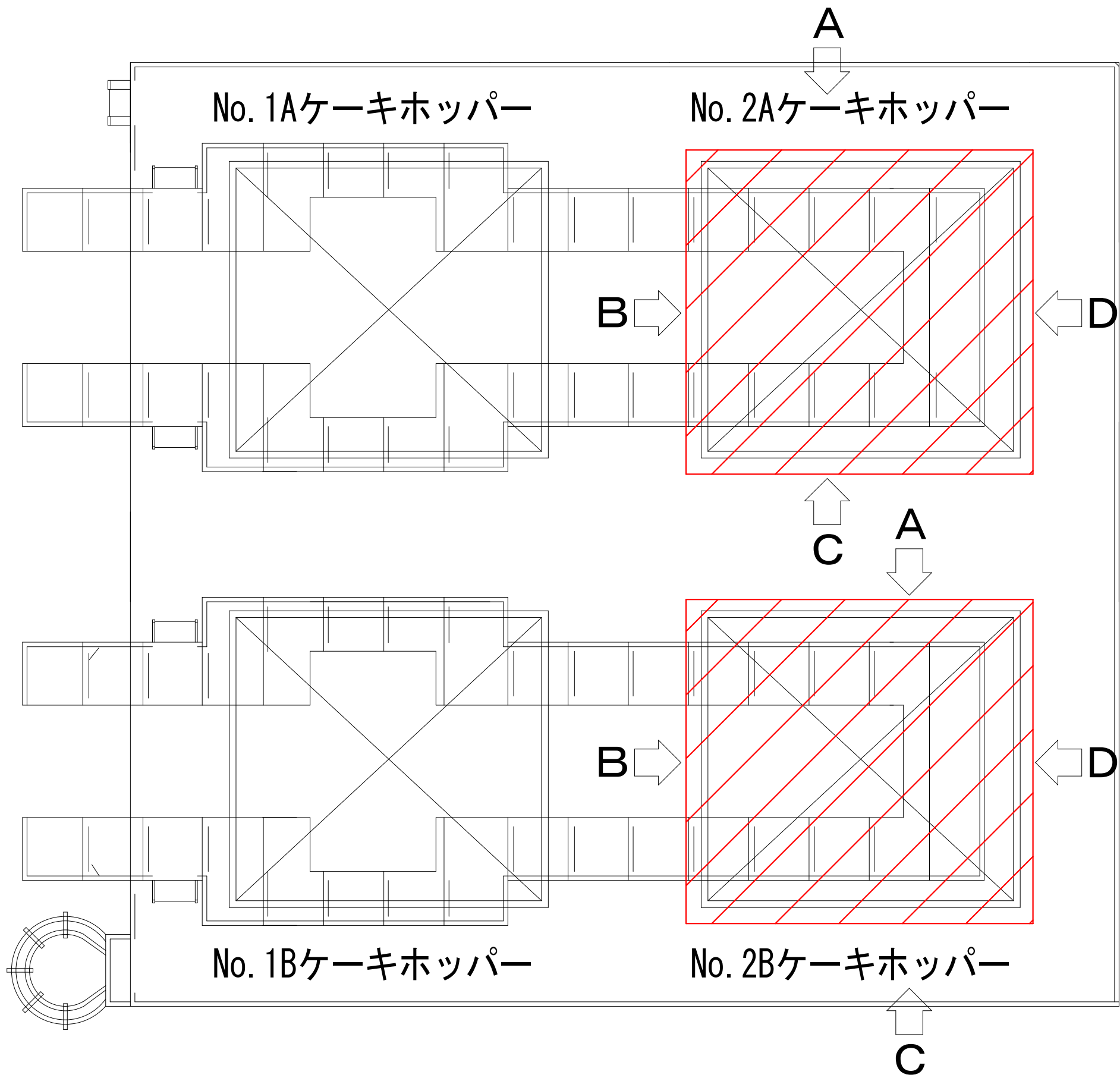
脱水ケーキ貯留ホッパー 平面図 A1:S=1/ 50 A3:S=1/100
