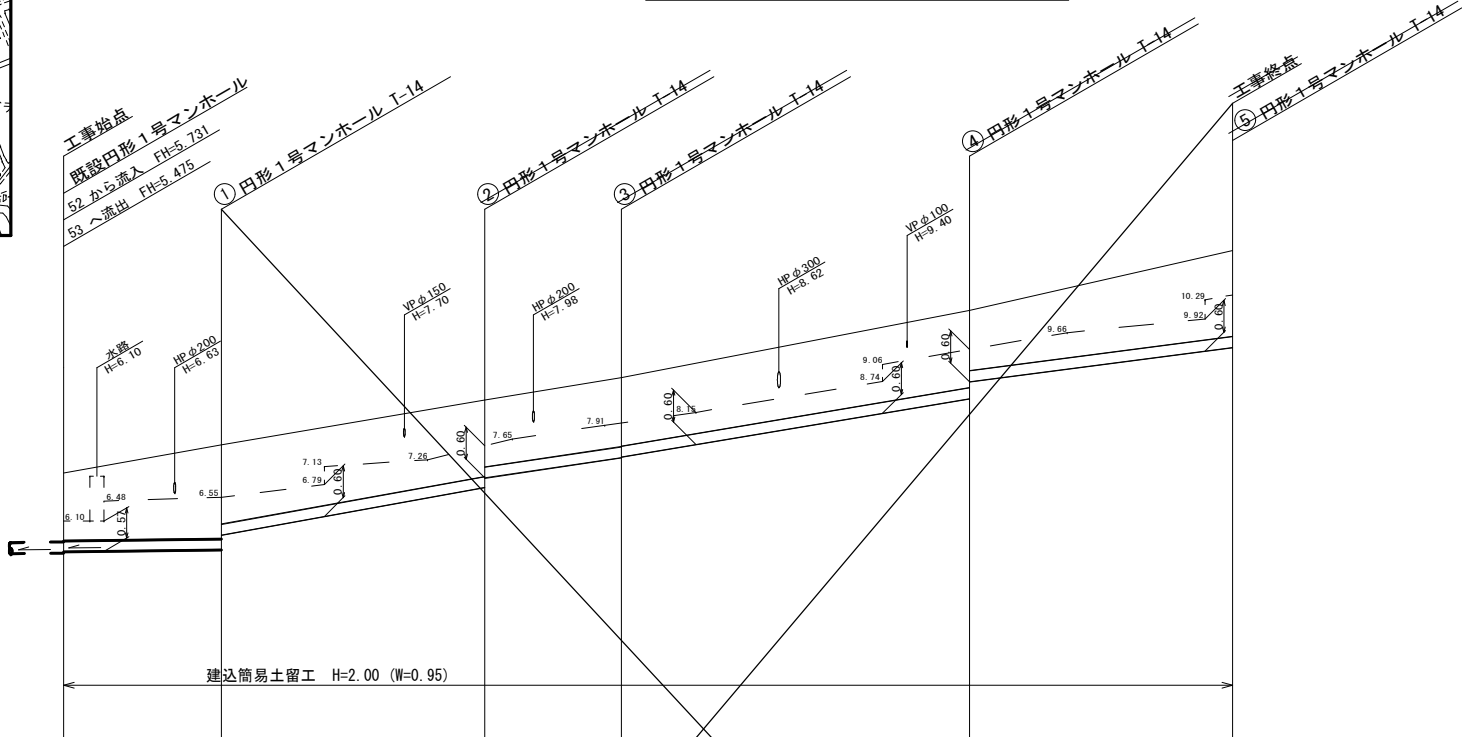
管渠埋設縦断面図
