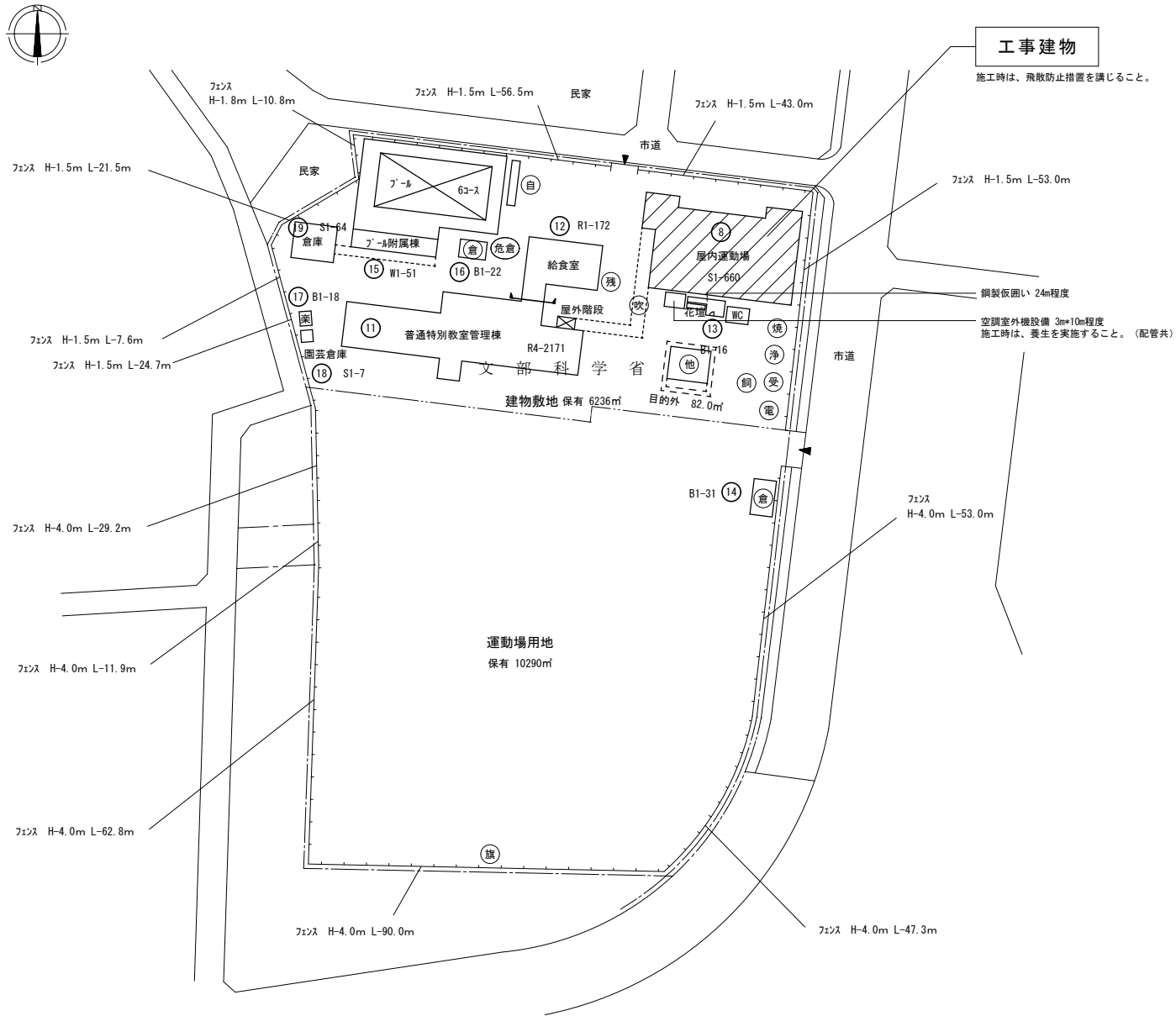
配置図 S=1/1500
