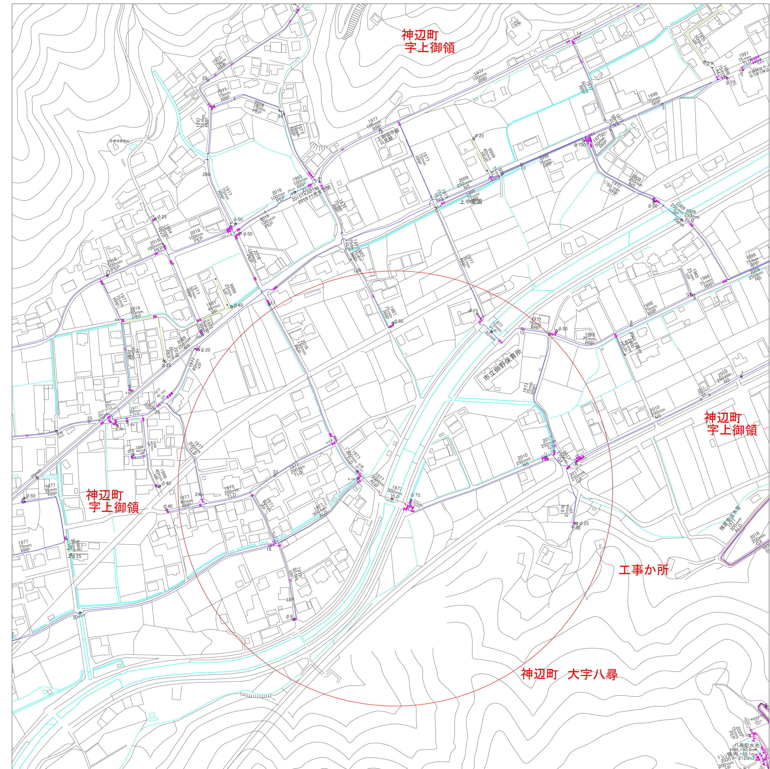
配管図 S=1/2500
