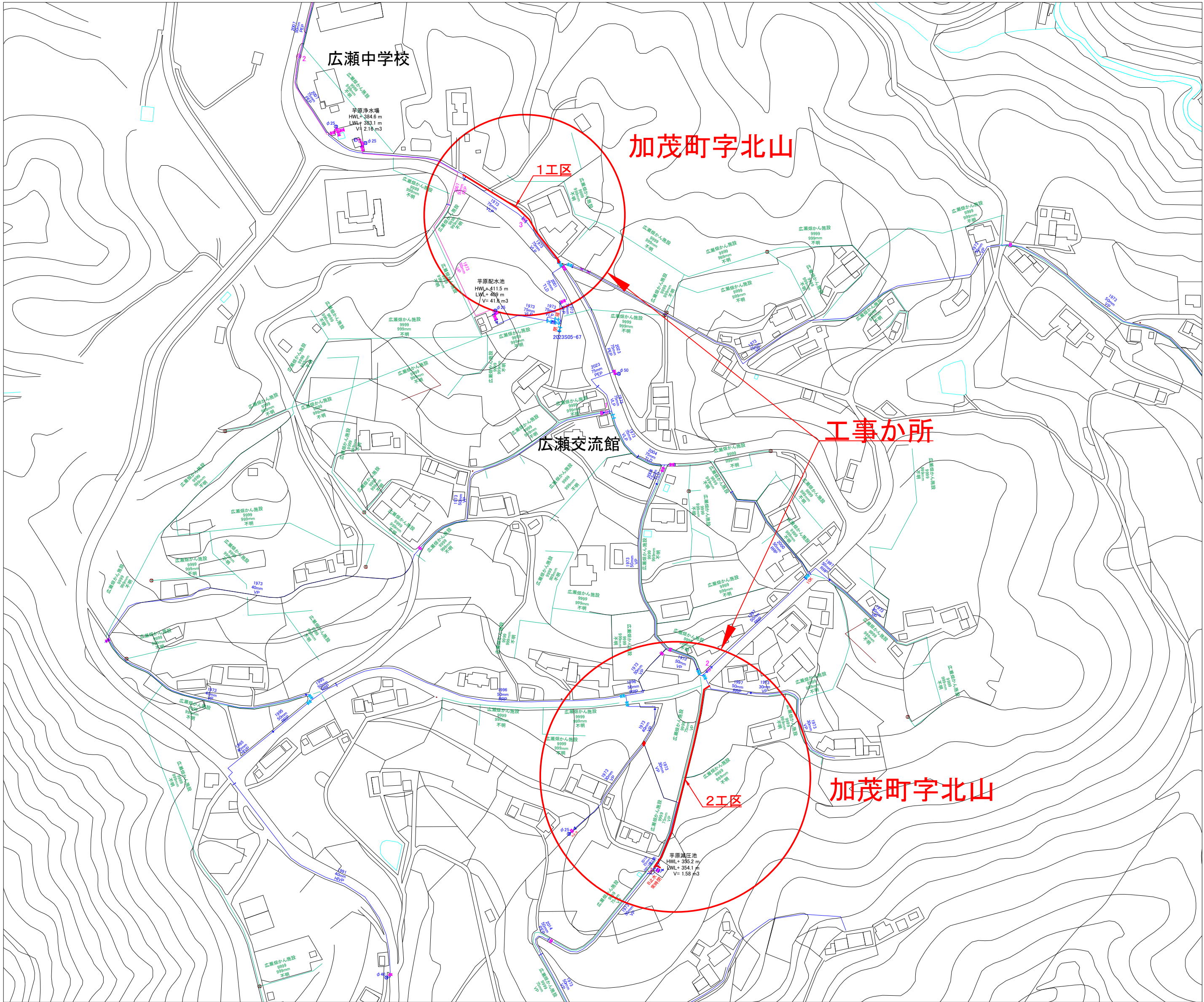
配 管 図 S=1:2500
