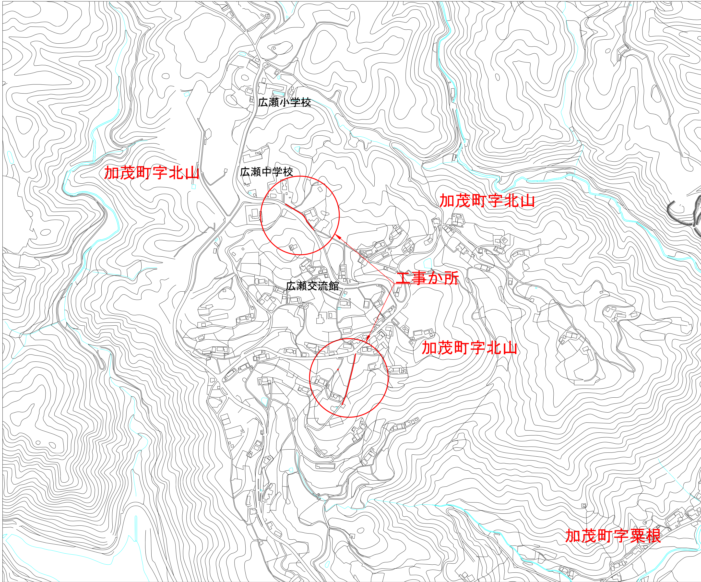
位 置 図 S=1:5000
