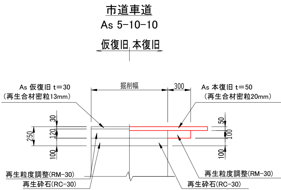
舗装復旧図 S=Non
