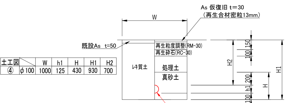
消火栓土工図
