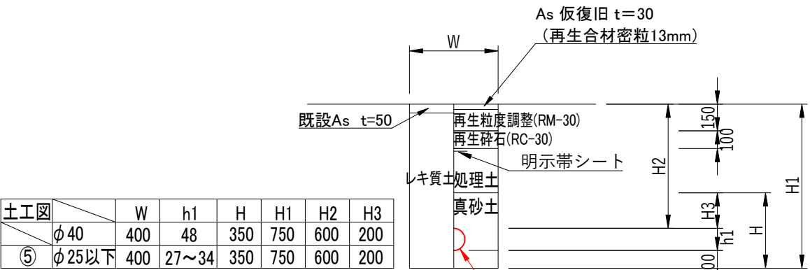
②PP土工図 (市道車道部)
