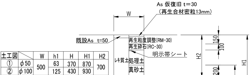
標準土工図 S=1/30 PEP土工図 (市道車道部)
