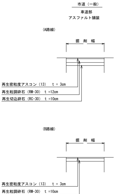
舗装復旧断面 S=1/50
