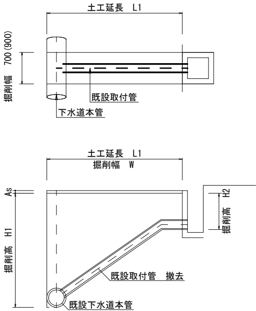
標準取付管撤去図
