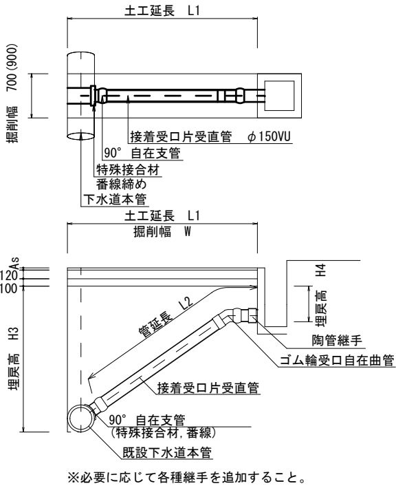
標準取付管埋設図
