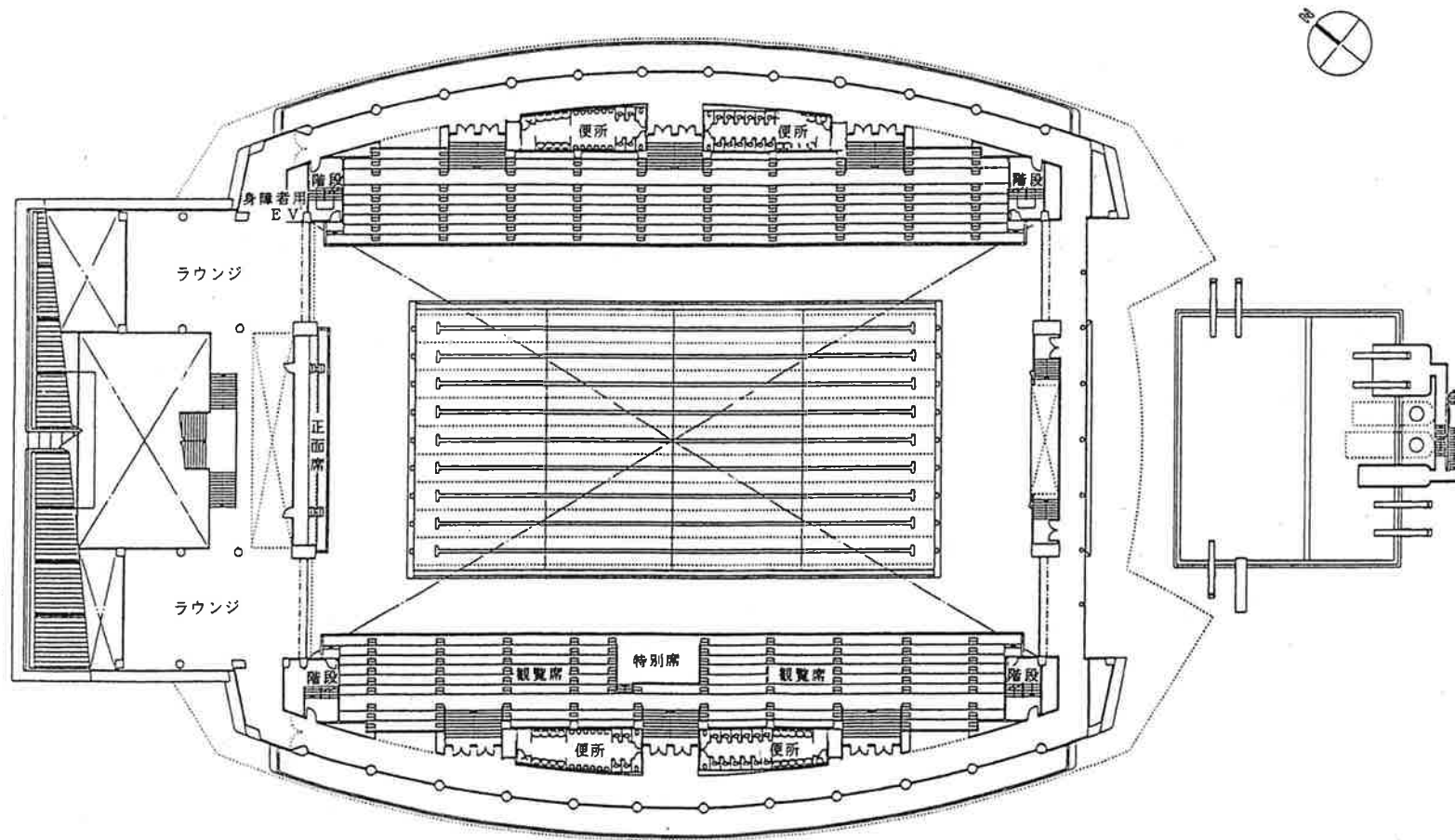
緑町公園屋内競技場（ローズアリーナ） 平面図 2F
