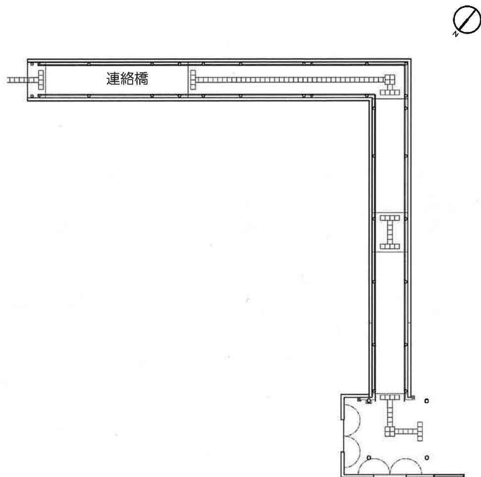
福山市緑町公園屋内競技場 2.5 m プール 連絡橋平面図
