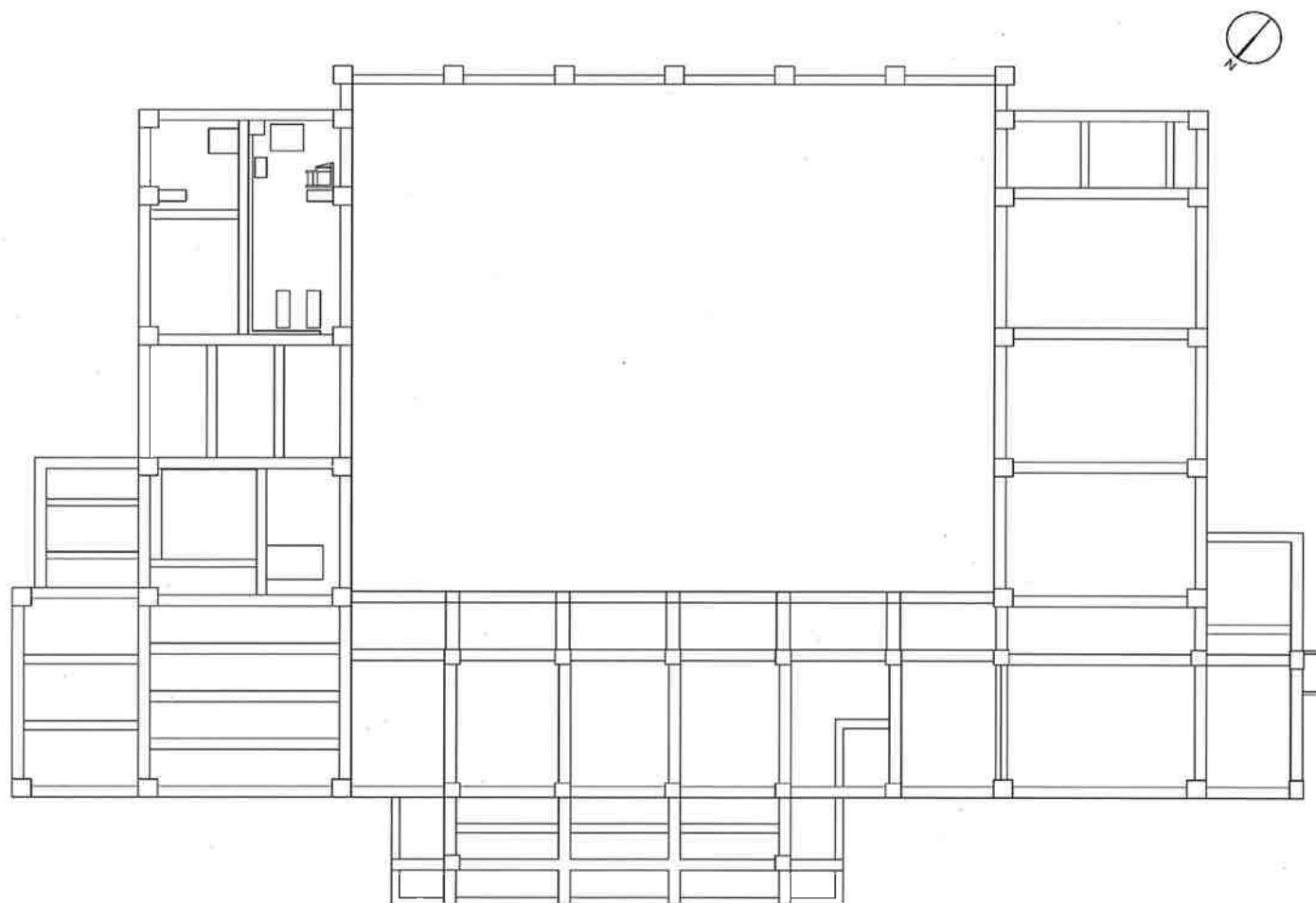
福山市緑町公園屋内競技場 25mプール 地下平面図
