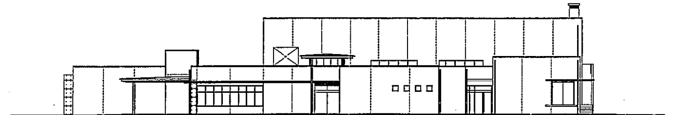
東側立面図
