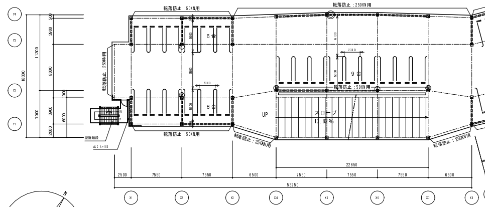
4 階平面図
