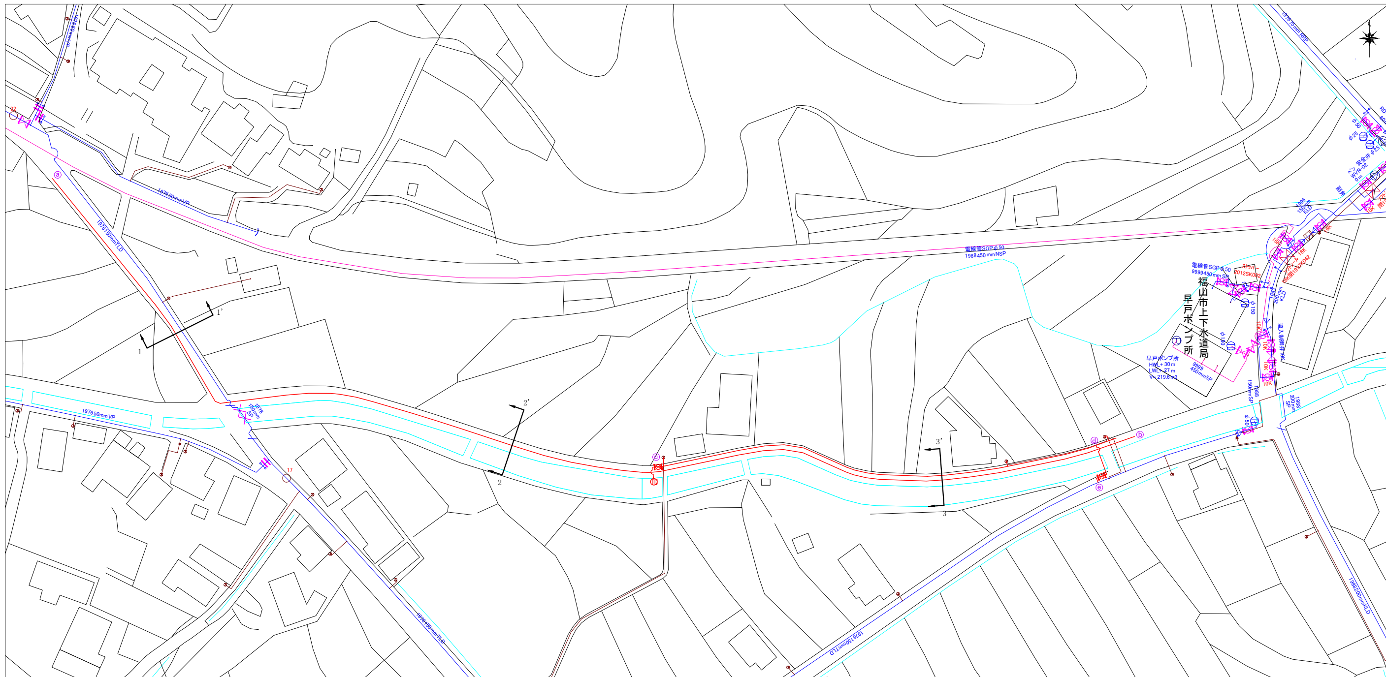
平面図 S=1/500
