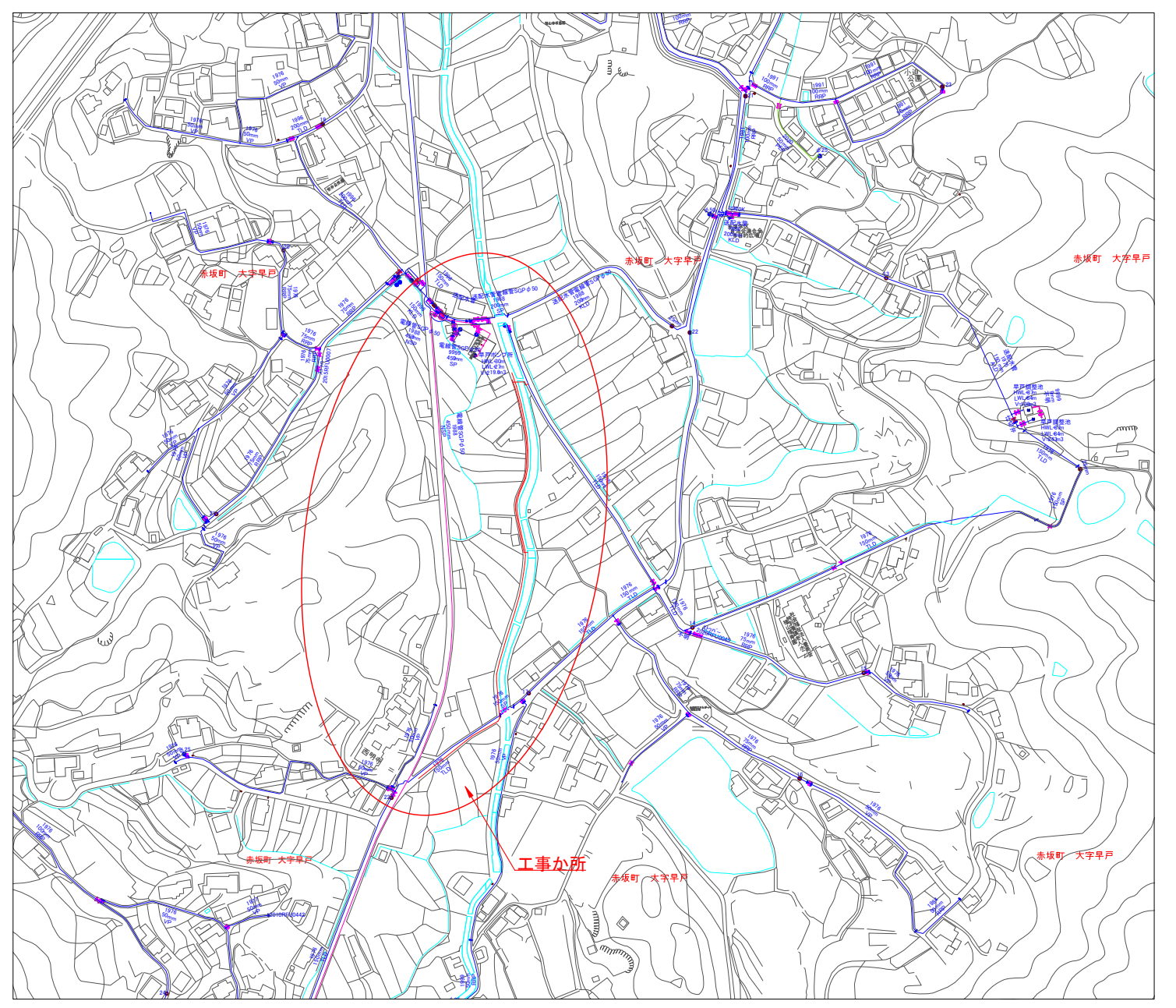
配管図 S=1/2,500
