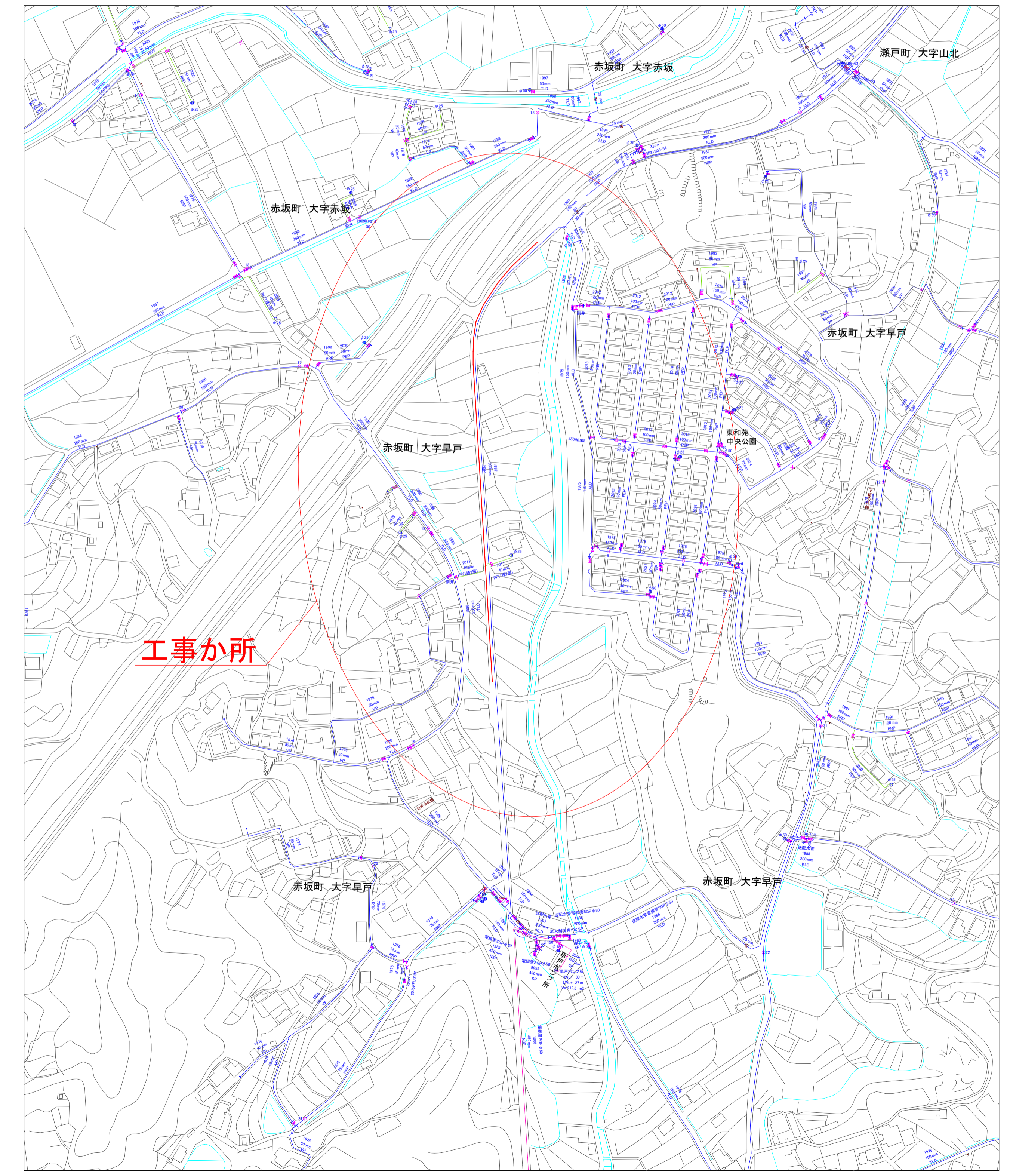
配管図 S=1/2,500
